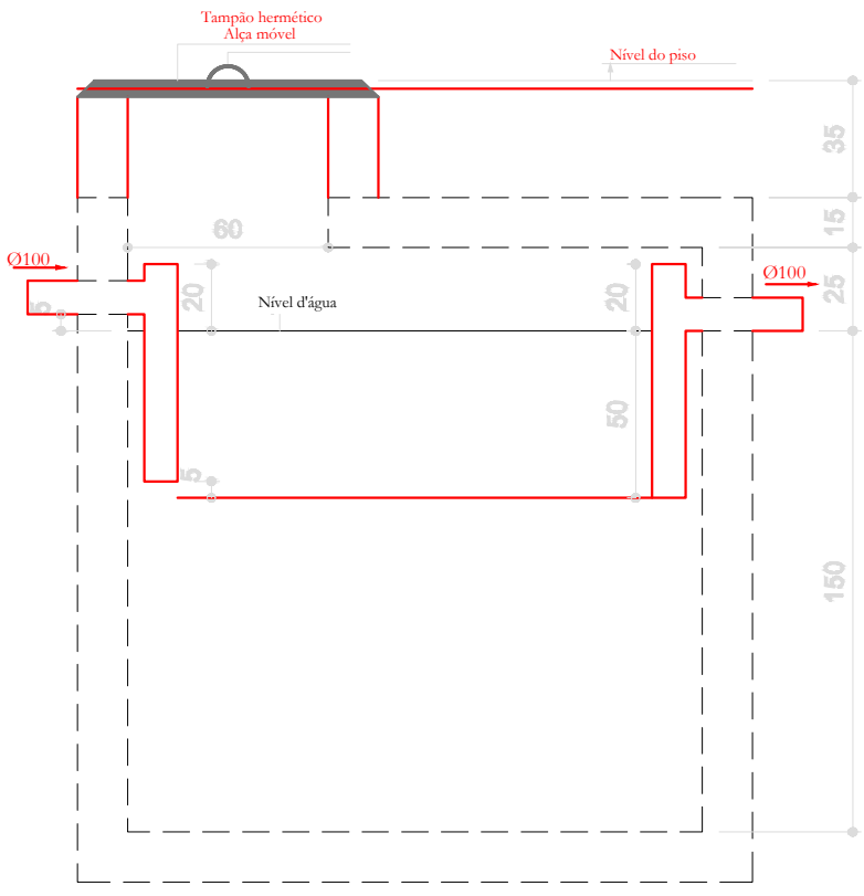
Tanque séptico Corte 1- ESC. 1:25
