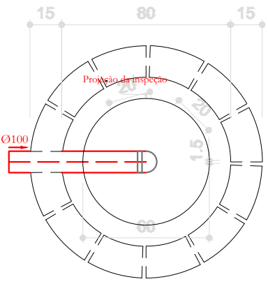
Sumidouro Planta baixa - ESC. 1:25
