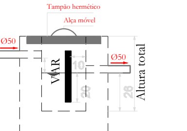
Caixa de gordura Corte 1- ESC. 1:25
