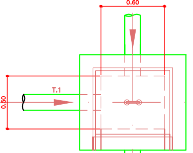
PLANTA ESC. 1:20
