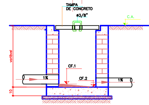
CORTE ESC. 1:20
