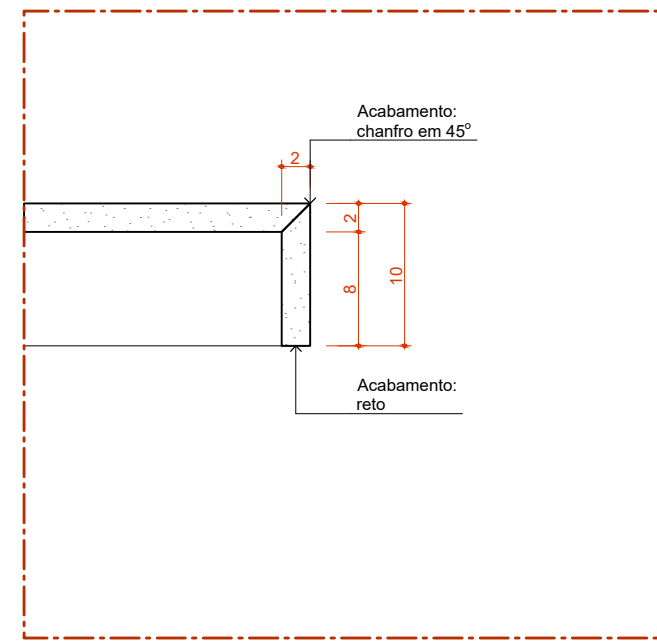
Det. B.P.b Bancada de Pedra Detalhe Saia
