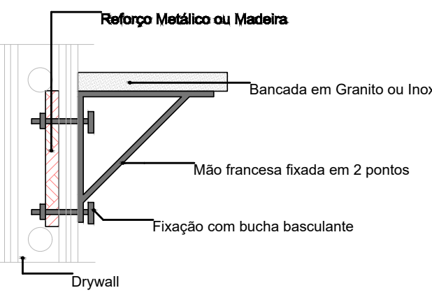
DETALHE 01: REFORÇO EM DRYWALL
