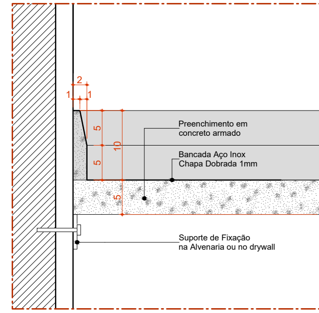
Det. B.I.c Bancada de Inox Detalhe Frontão - Área Secca
