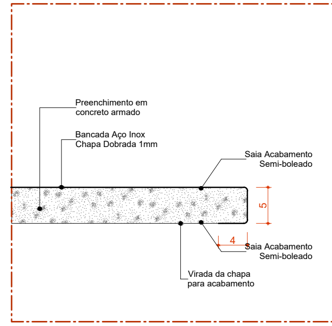
Det. B.I.d Bancada de Inox Detalhe Saia - Área secca
