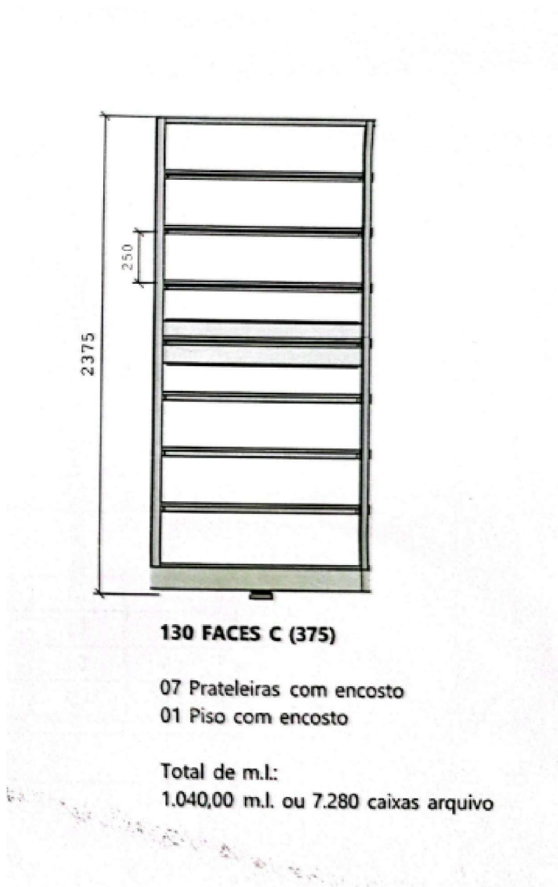
Detalhamento Prateleiras Sem Escala
