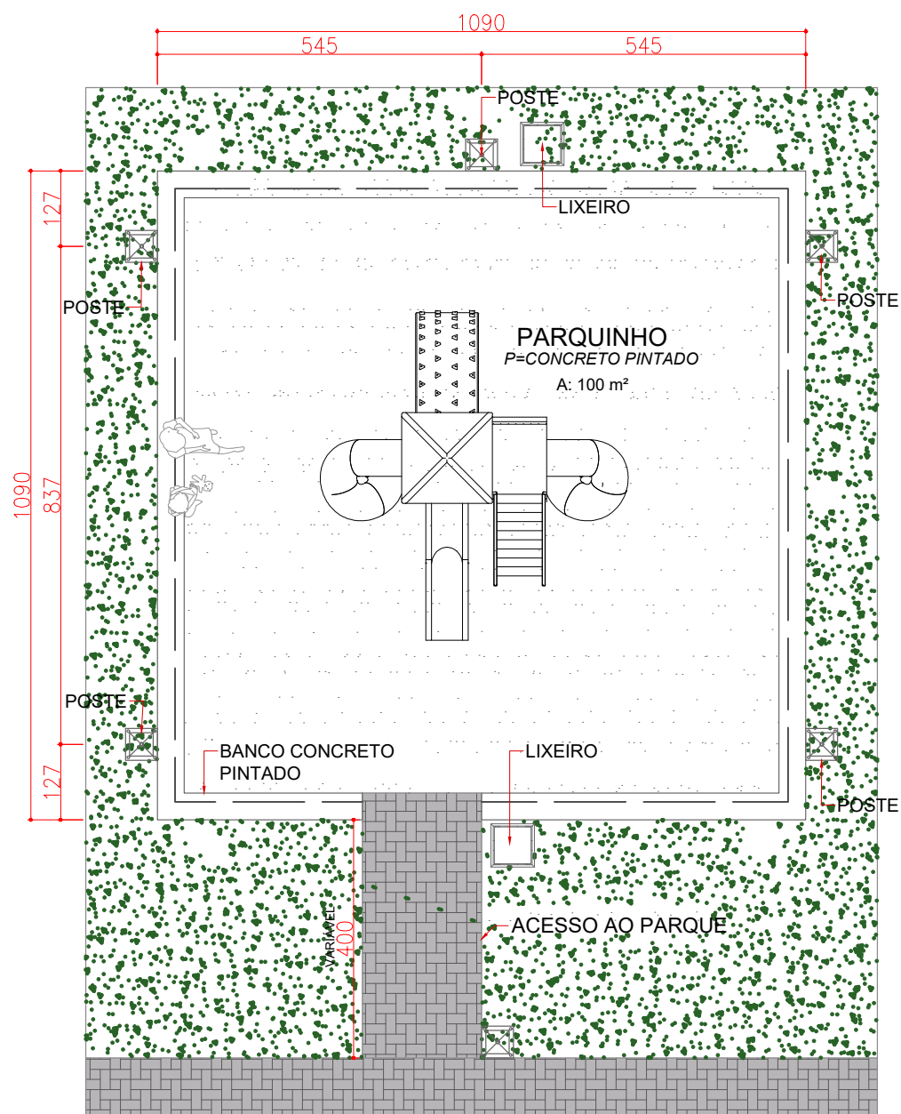
PLANTA BAIXA ESC.:.....1/100
