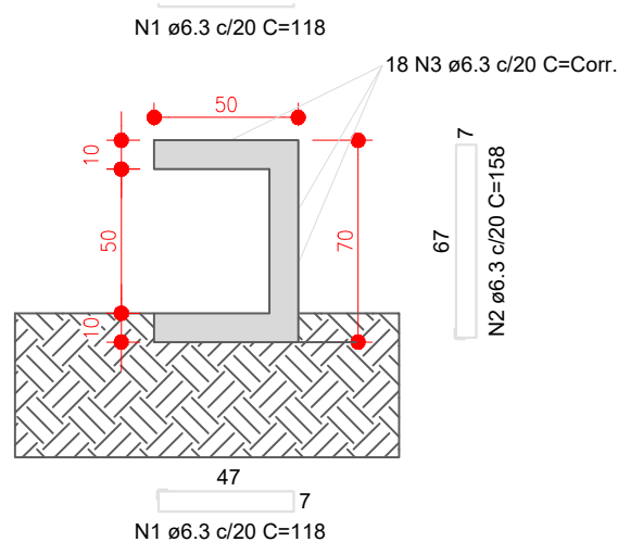
CORTE A-A ESC.:.....sem
