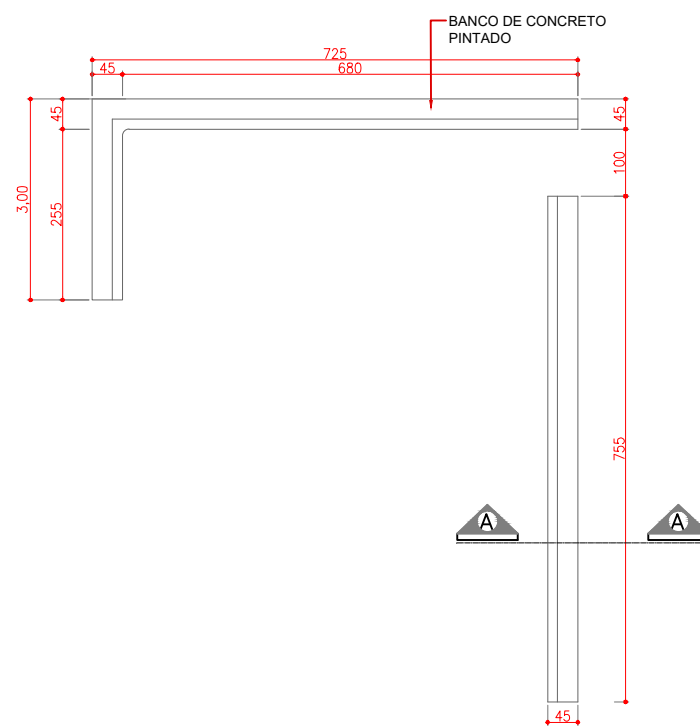
DETALHAMENTO DO BANCO ESC.:.....1/100
