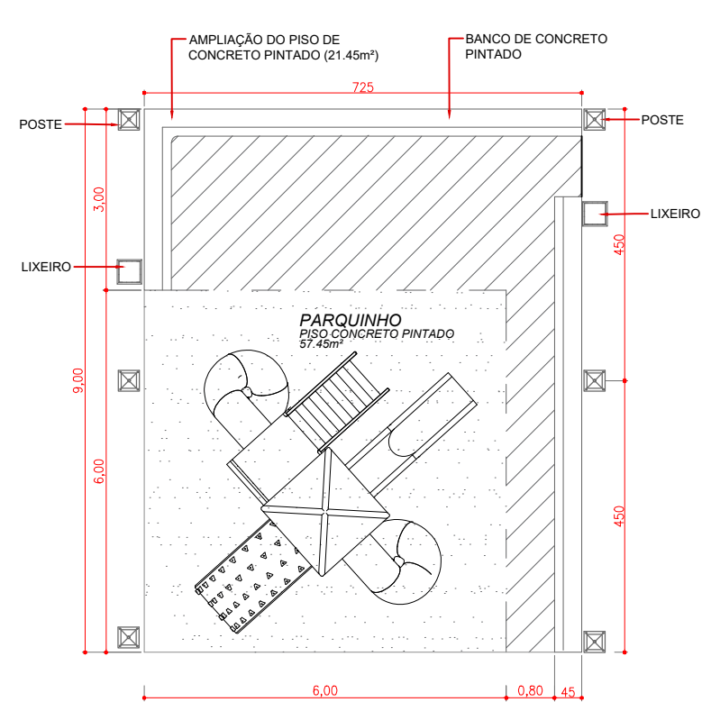
PLANTA BAIXA ESC.:.....1/100
