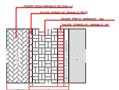
DET. BORDA DAS CALÇADAS E ARRANJO PARA COLOCAÇÃO DE PAVER
