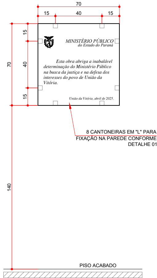
ELEVÇÃO ESCALA 1: 20
