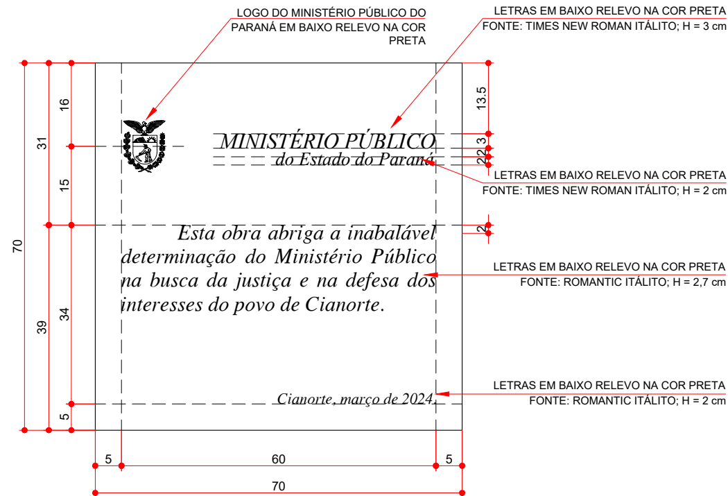
VISTA PLACA ESCALA 1:10
