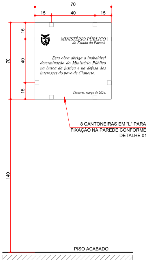
ELEVÇÃO ESCALA 1: 20
