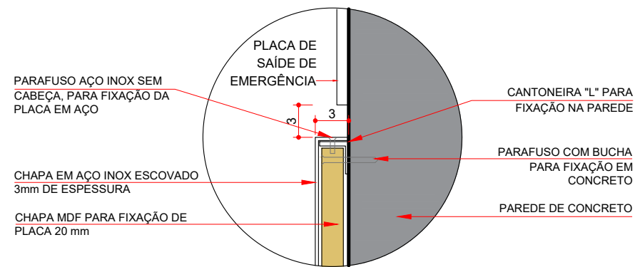
DETALHE 01 ESCALA 1: 5
