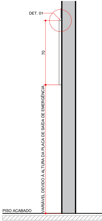
CORTE ESCALA 1: 20
