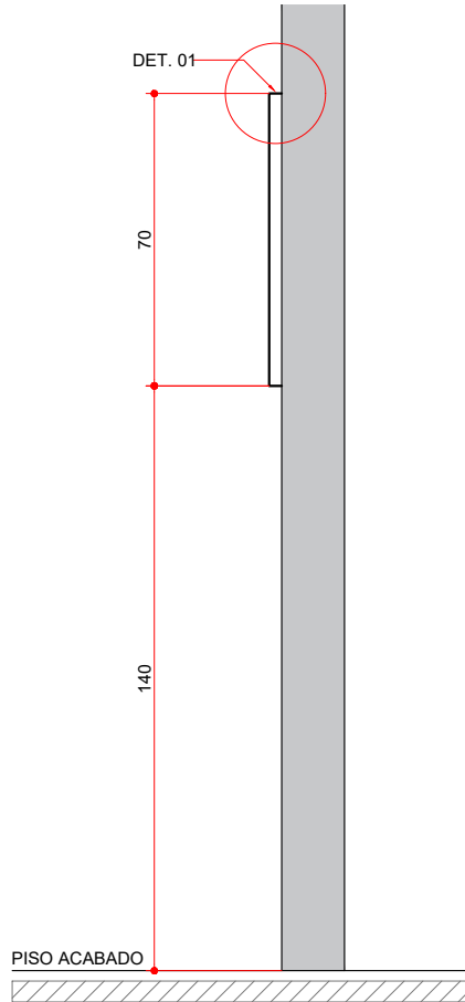
CORTE ESCALA 1: 20
