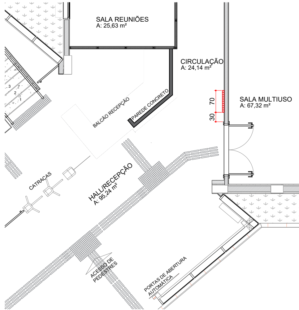
LOCALIZAÇÃO TÉRREO ESCALA 1:75
