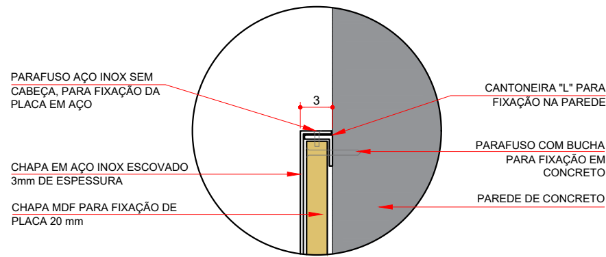
DETALHE 01 ESCALA 1: 5
