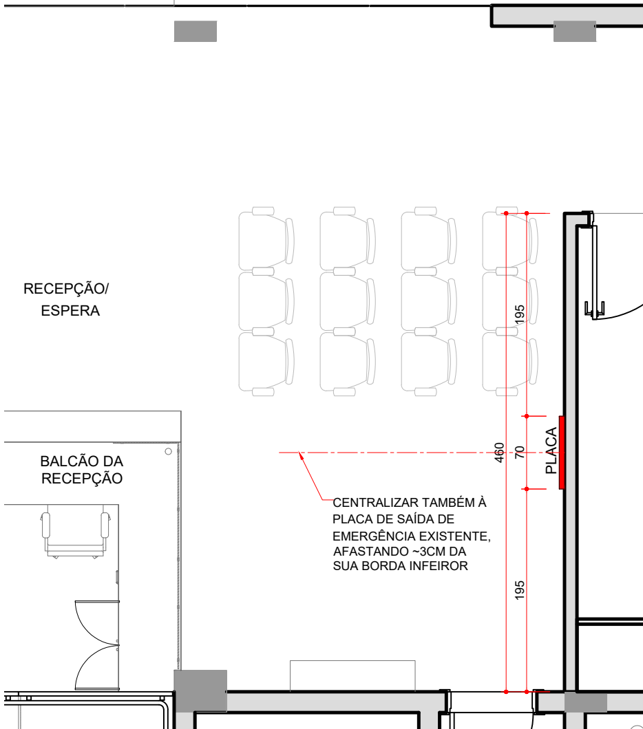
LOCALIZAÇÃO TÉRREO ESCALA 1/50
