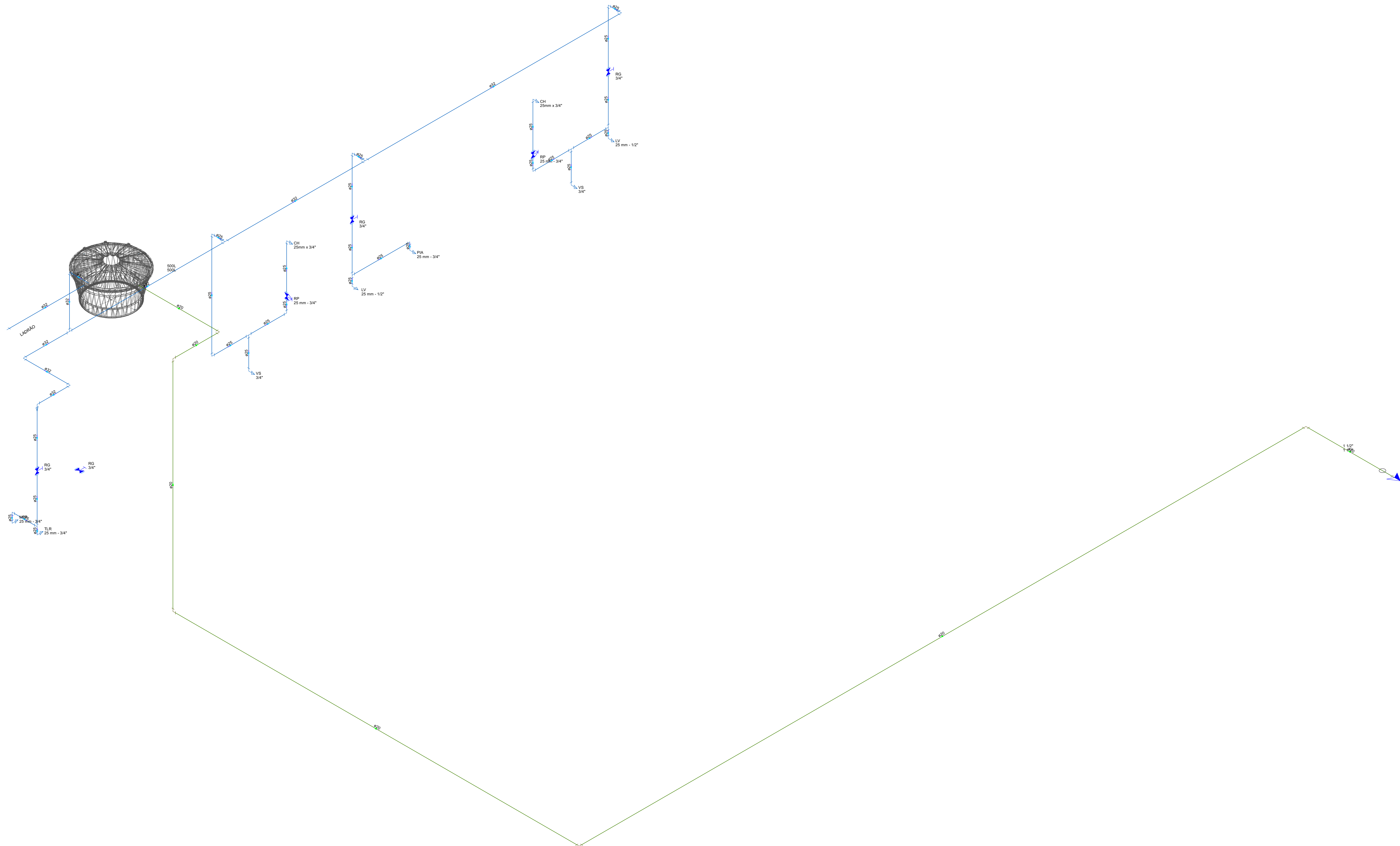
Esquema isométrico Hidráulico Escala 1:25
