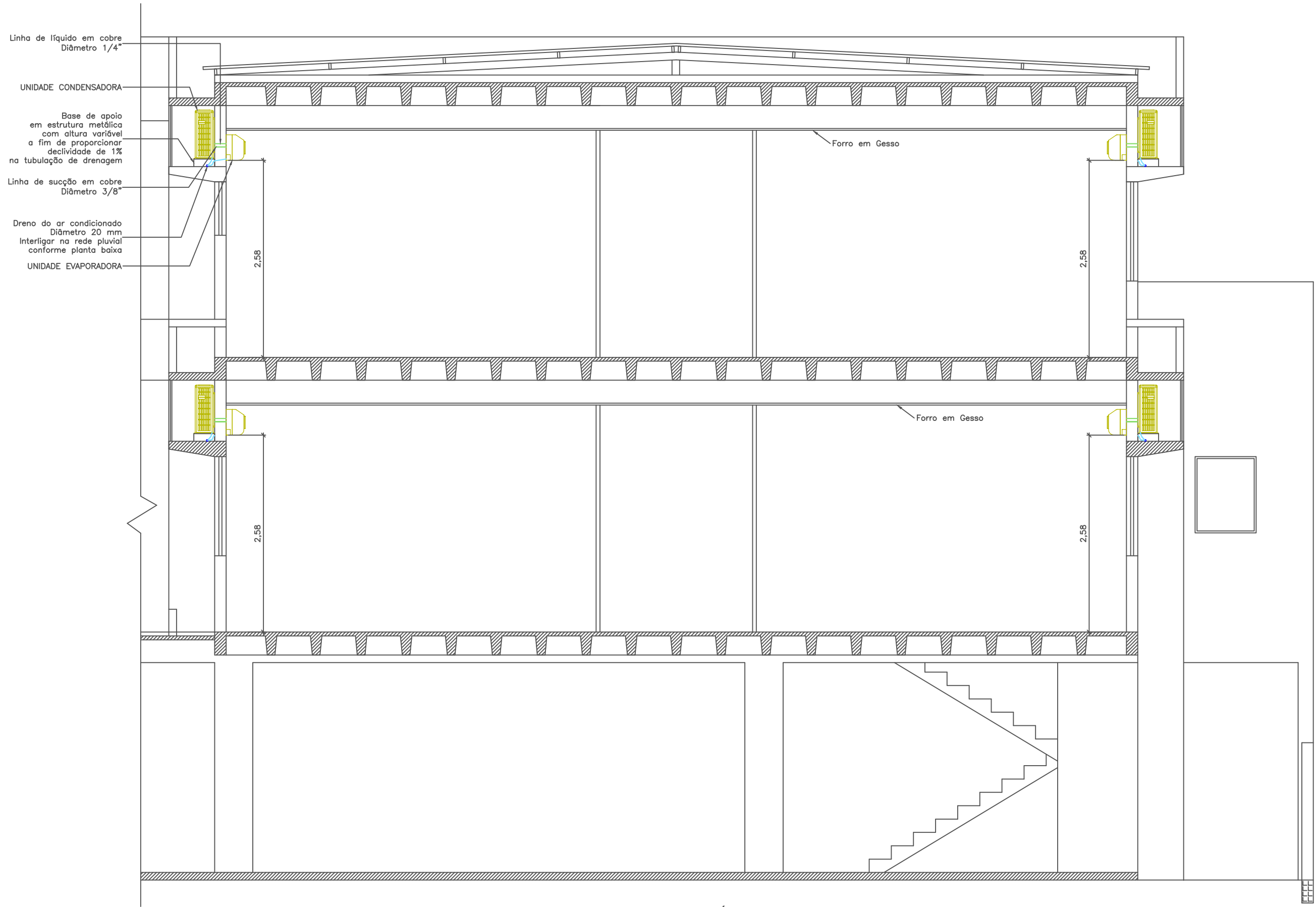
CORTE ESQUEMÁTICO DA INSTALAÇÃO DOS CLIMATIZADORES NAS SALAS DOS VEREADORES Esc.:1:50
