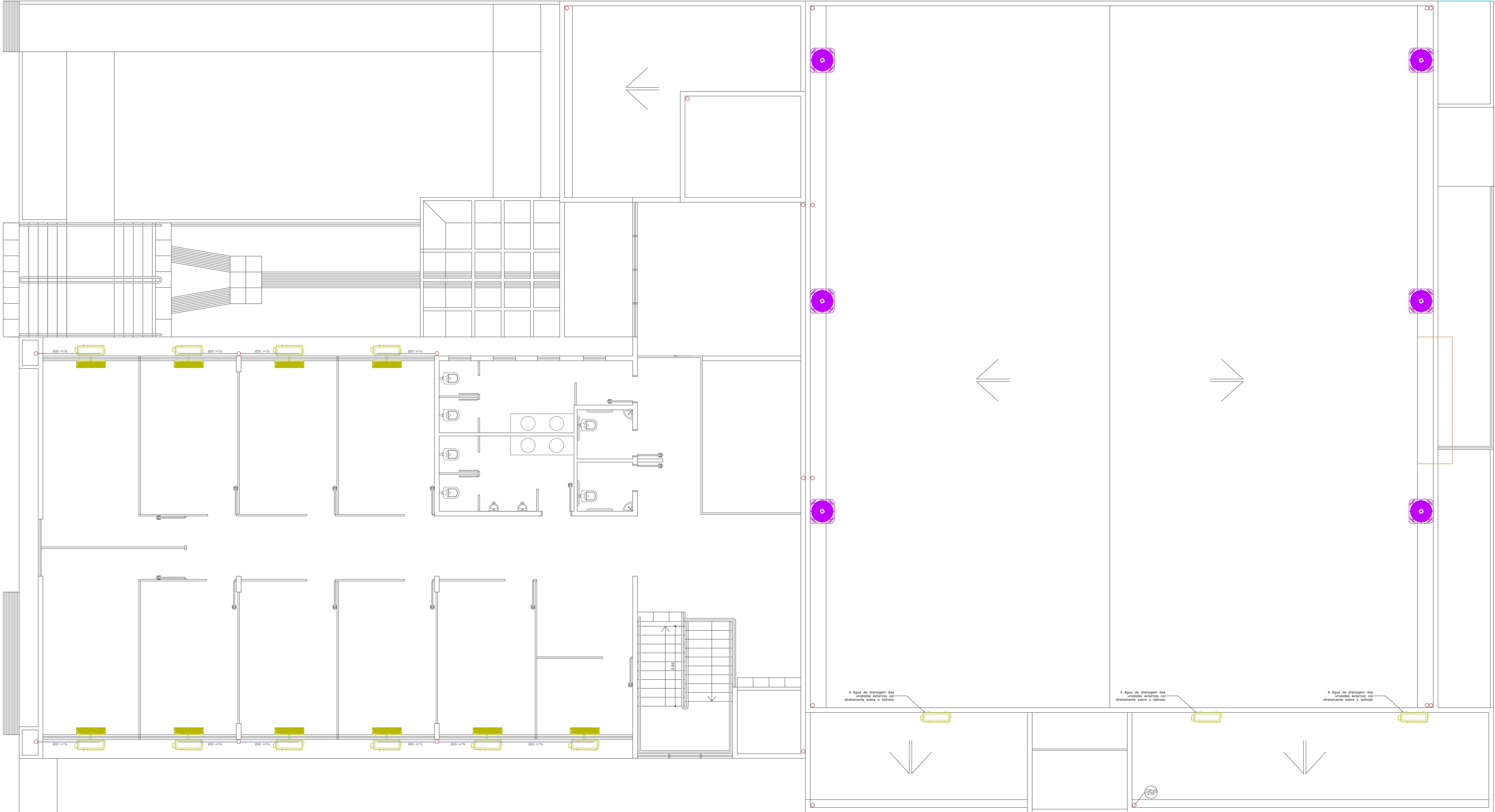
PLANTA BAIXA 1º PAVIMENTO Esc: 1:50
