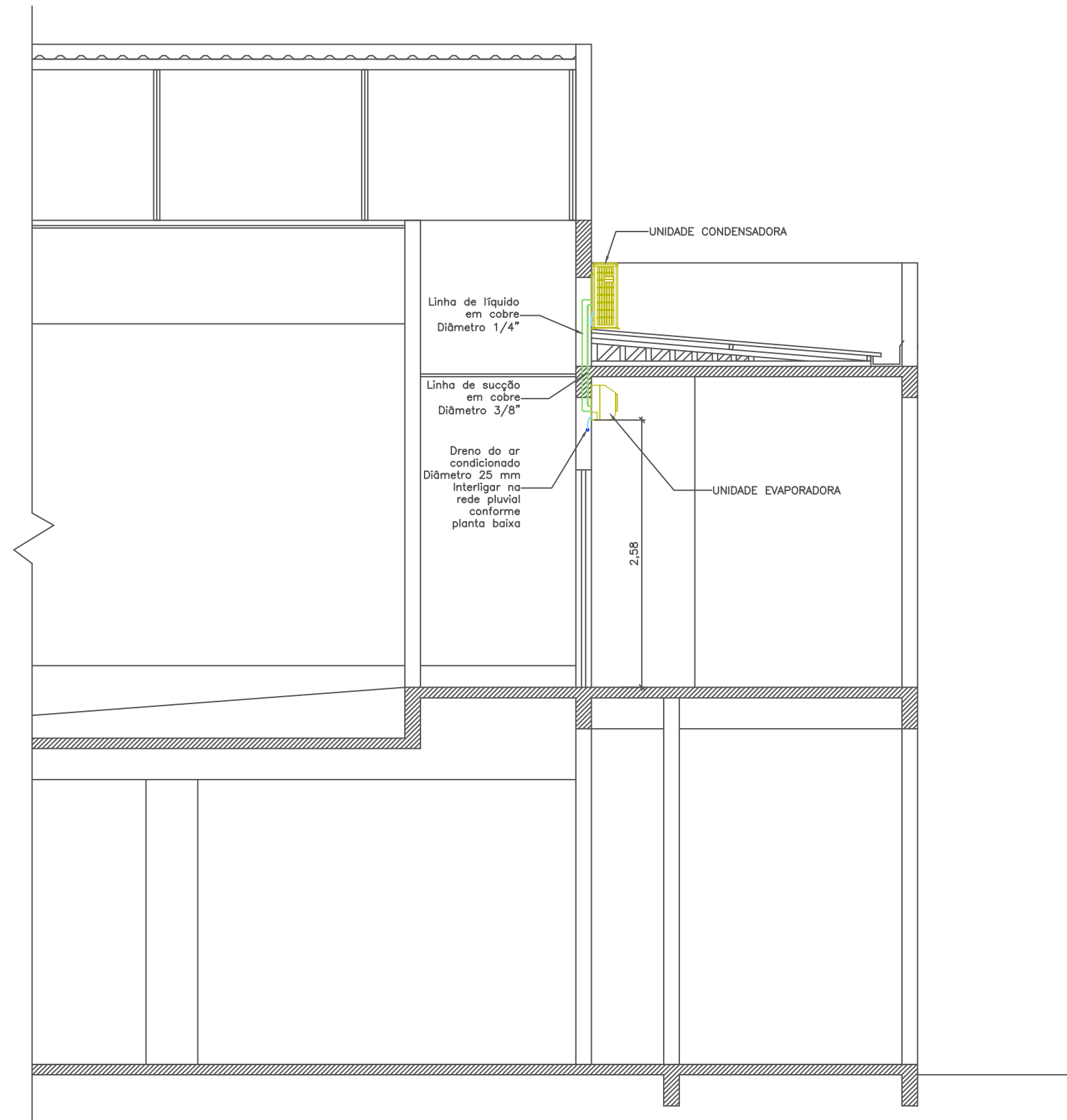
CORTE ESQUEMÁTICO DA INSTALAÇÃO DOS CLIMATIZADORES NAS SALAS DO PRESIDENTE, COMISSÕES E REUNIÕES Esc.:1:50
