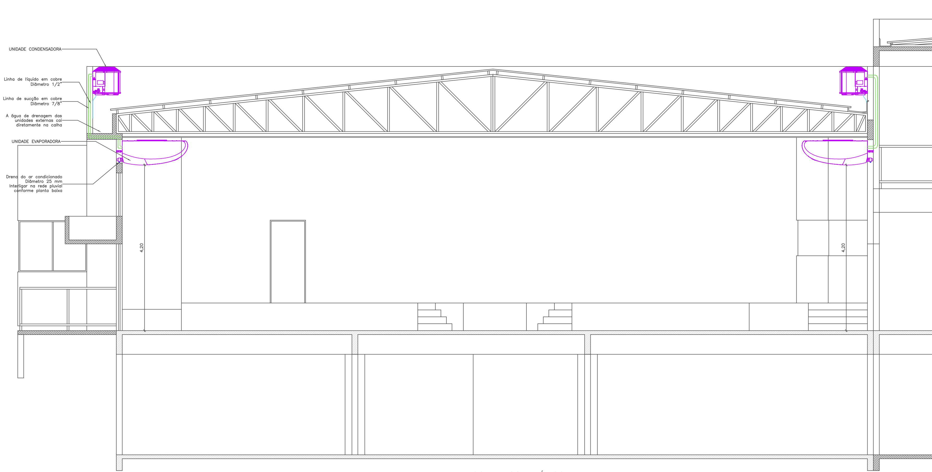
CORTE ESQUEMÁTICO DA INSTALAÇÃO DOS CLIMATIZADORES NO AUDITÓRIO Esc.:1:50
