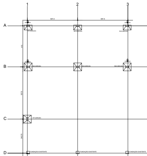
Planta estrutural sapatas Escala: 1:75
