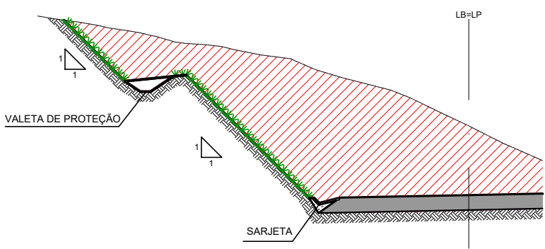
ARRASAMENTO ENLEIVAMENTO - PLANTIO DE GRAMA EM PLACAS
