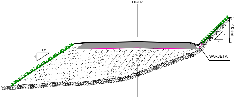
TALUDES DE ATERRO OU TALUDE DE CORTE COM ALTURA MENOR QUE 0,5m ENLEIVAMENTO - PLANTIO DE GRAMA EM PLACAS
