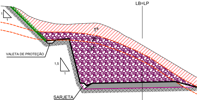
TALUDES DE CORTE COM 3ª CATEGORIA (ROCHA) HIDROSSEMEADURA
