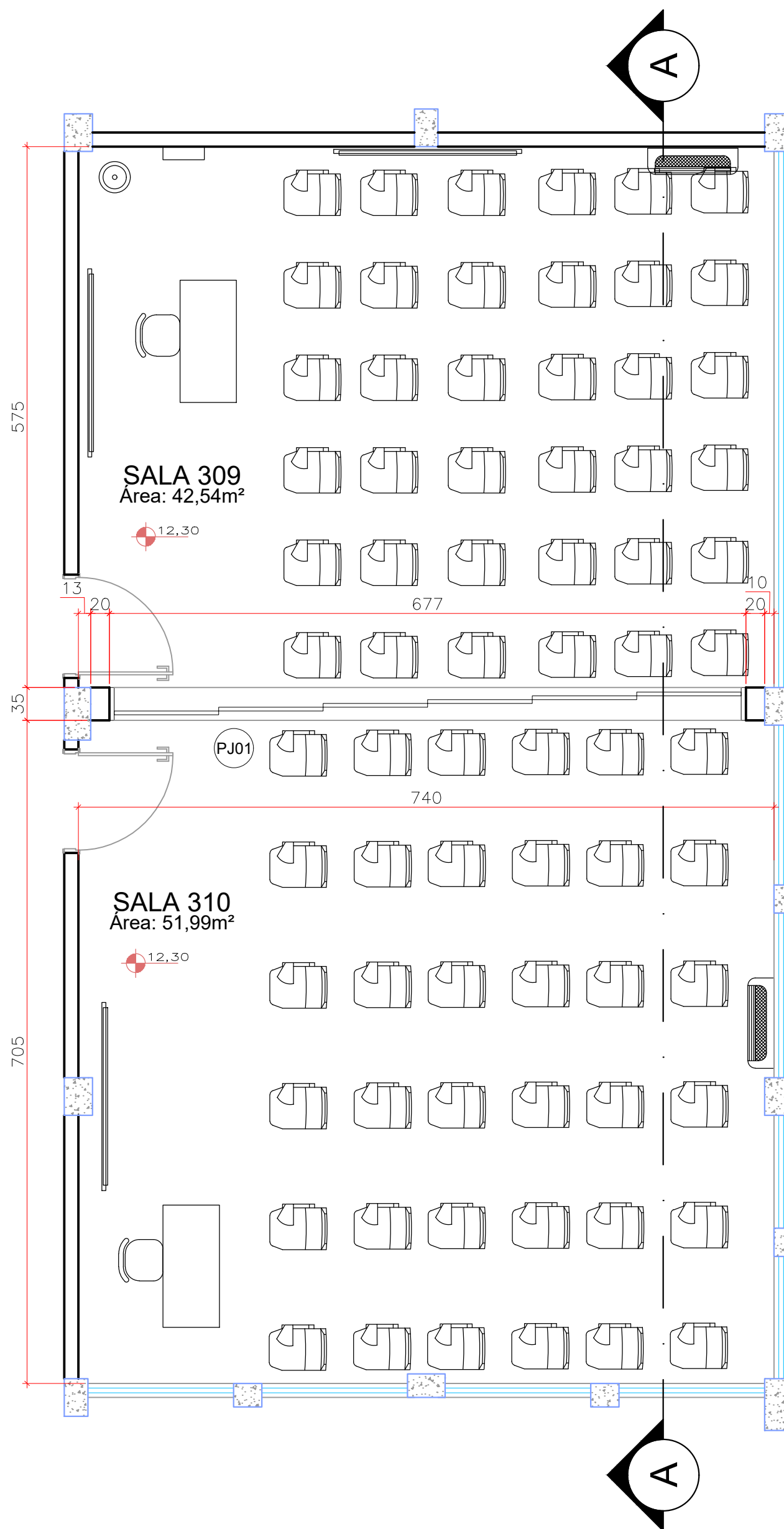
PLANTA BAIXA - SALAS 309 E 310 CEAPAC ESCALA - 1:50 - OPÇÃO 02 LAYOUT A: 94,53m²
