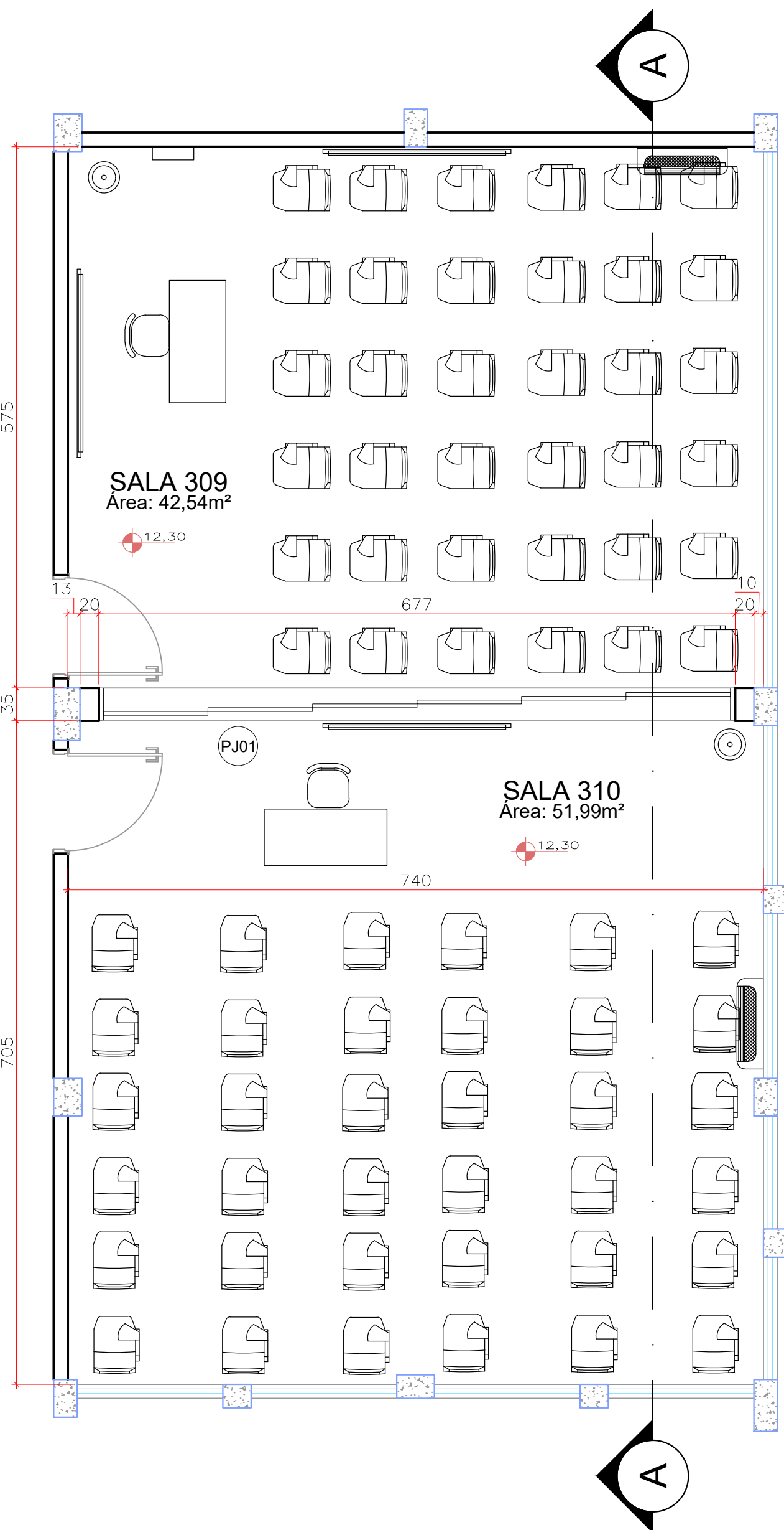
PLANTA BAIXA - SALAS 309 E 310 CEAPAC ESCALA - 1:50 - OPÇÃO 01 LAYOUT A: 94,53m²
