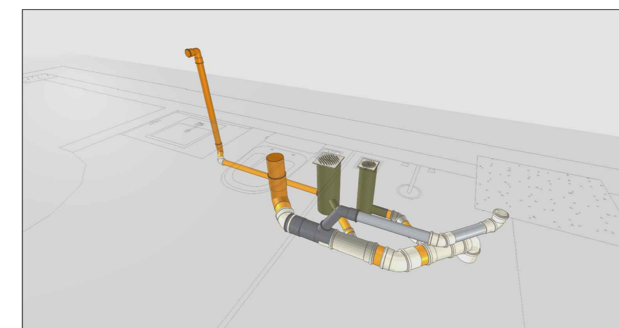
DETALHE TQ1 Sem escala
