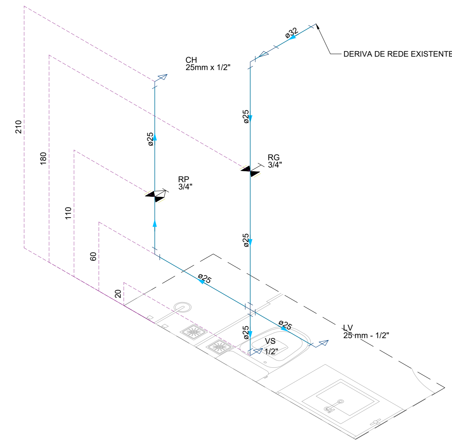
DETALHE HID-3 1:25
