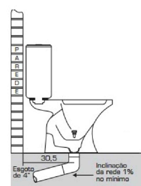
DETALHE Vaso Sanitário caixa acoplada Sem escala
