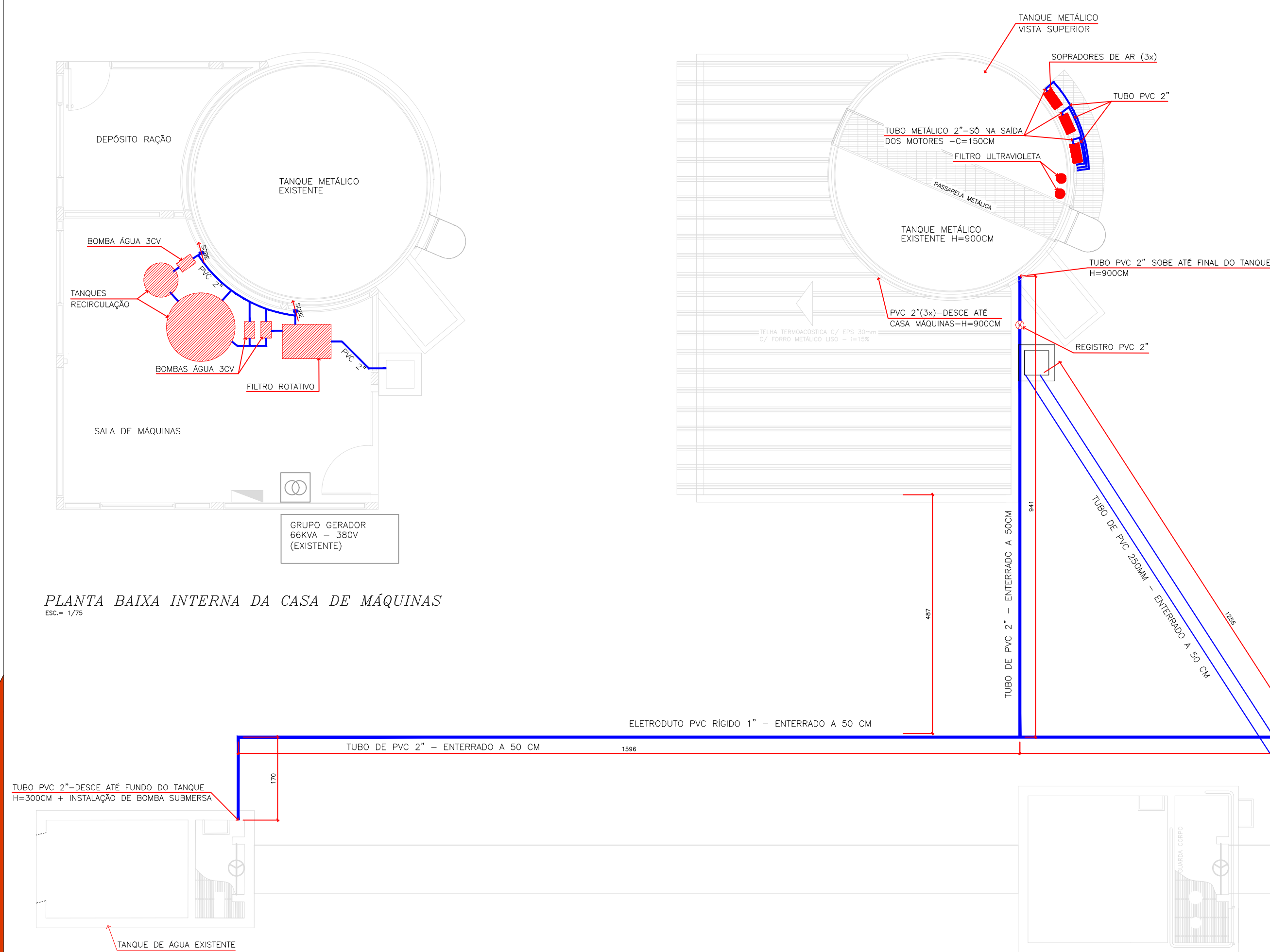
PLANTA BAIXA GERAL Esc. 1/16
