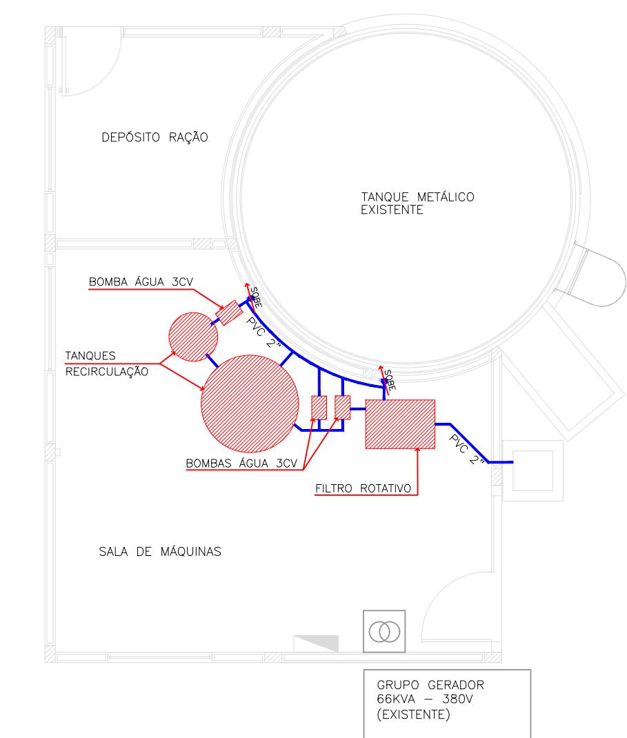
PLANTA BAIXA INTERNA DA CASA DE MÁQUINAS Esc. 1/16
