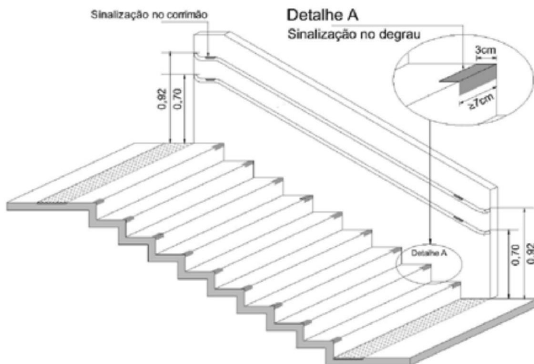
Figura 09: Esquema genérico do corrimão e sinalização em escada conforme NBR 9050-2020.
