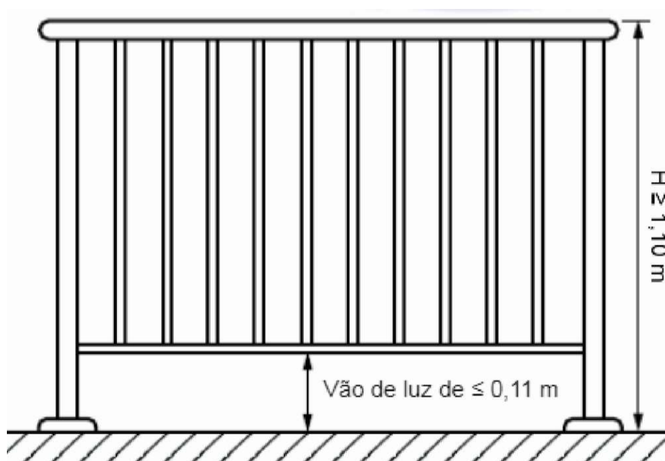
Figura 10: Esquema genérico do guarda-corpo conforme NBR 14718-2019.
