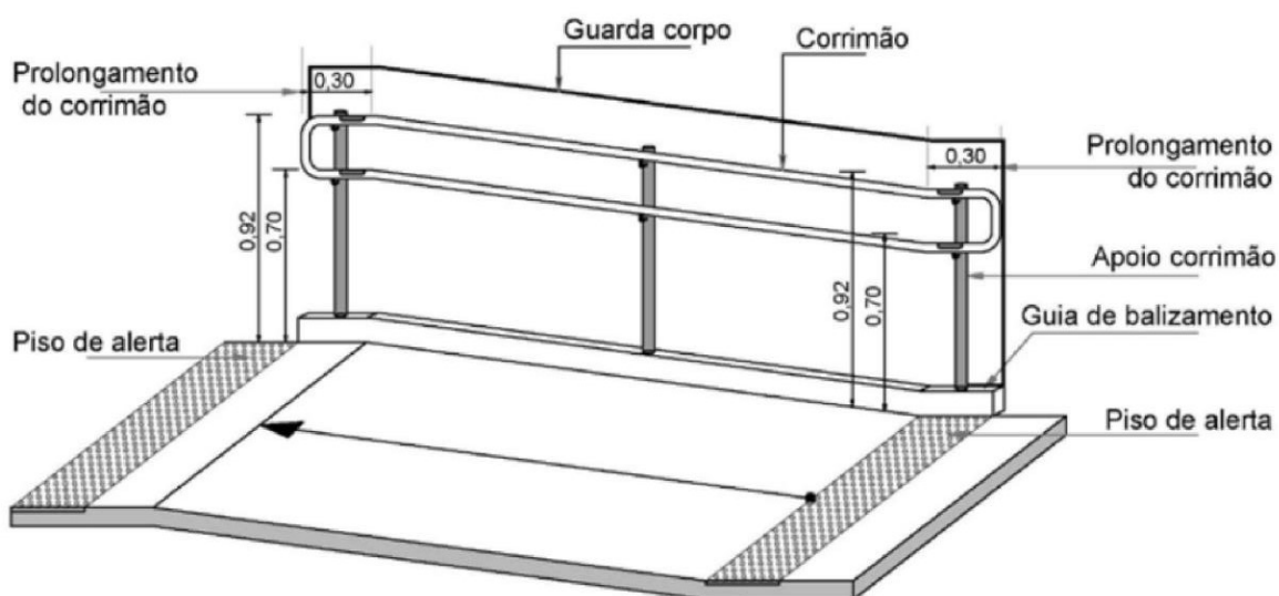
Figura 08: Esquema genérico do corrimão em rampa conforme NBR 9050-2020.
