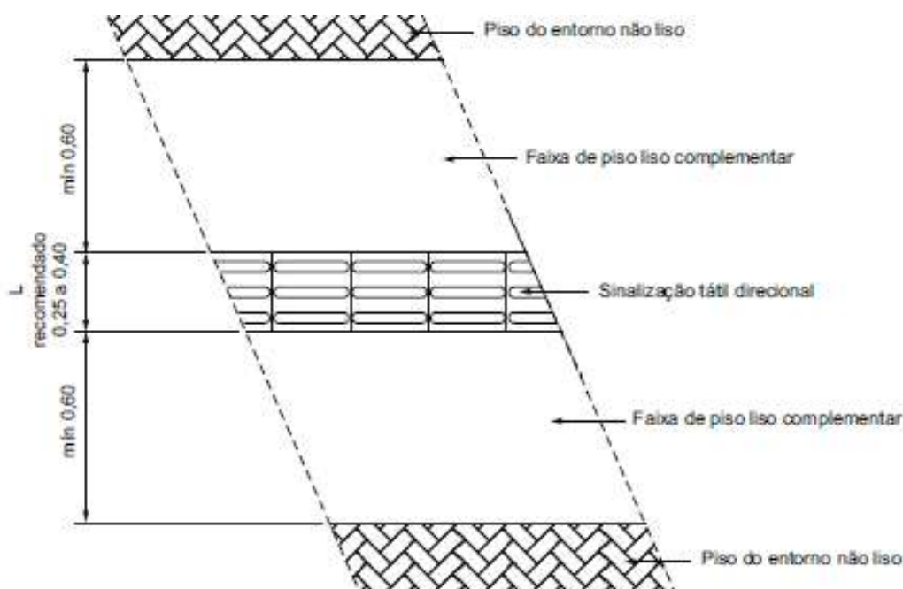
Figura 02: Piso tátil e direcional centralizado no passeio.
