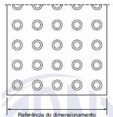
Figura 01: piso tátil direcional.
