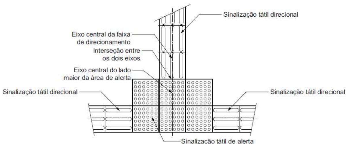
Figura 07: Piso de alerta e direcional unidos na mudança de direção.
