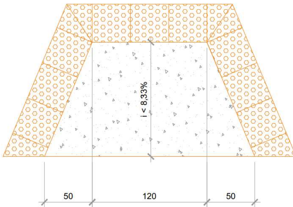
Figura 12: Detalhamento das rampas em concreto, medidas em centímetros.
