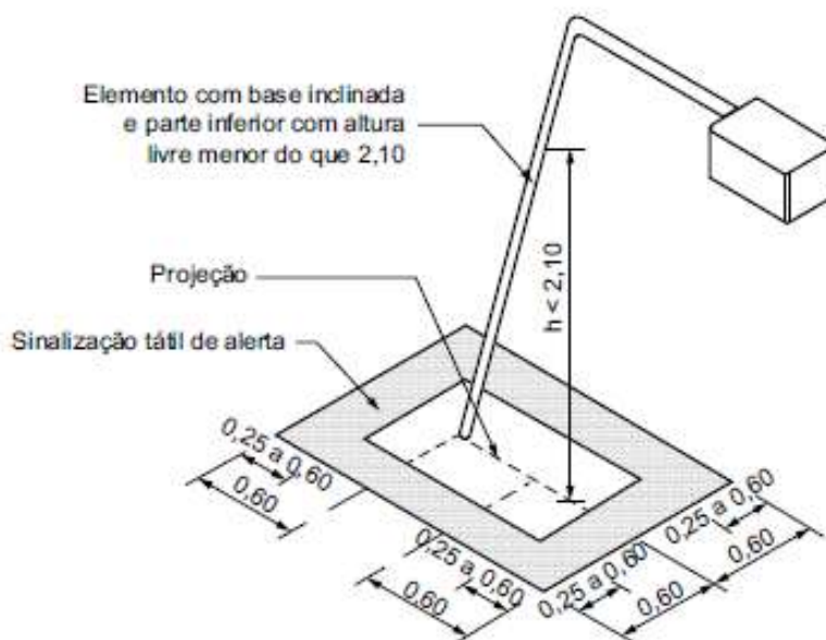
Figura 04: bloco intertravado de concreto tipo paver de alerta entorno de obstáculo para advertir o indivíduo.
