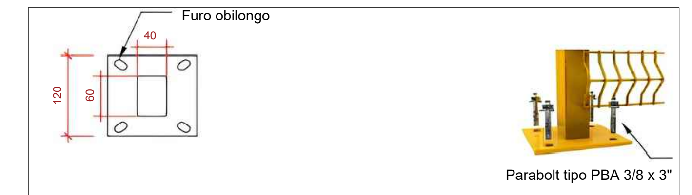
DETALHE 3-B Poste com base parafusada Sem escala
