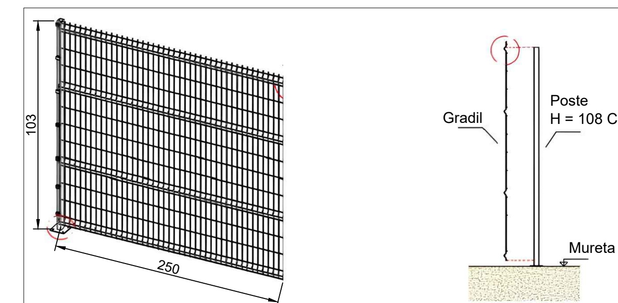
DETALHE 3-A Poste com base parafusada Sem escala
