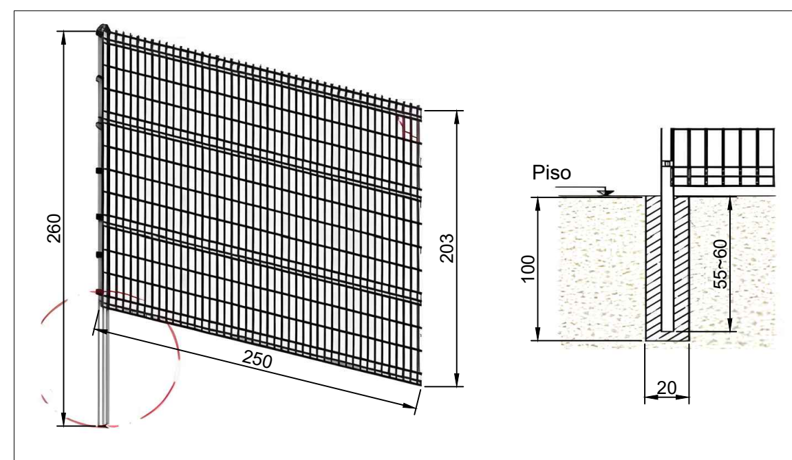
DETALHE 1 Poste com base concretada Sem escala
