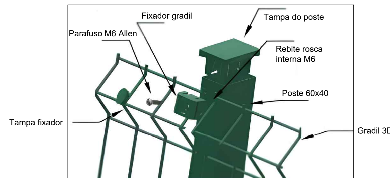
DETALHE 2 Fixação do gradil Sem escala
