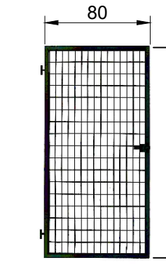
DETALHE 4 Porta de gradil genérica Sem escala
