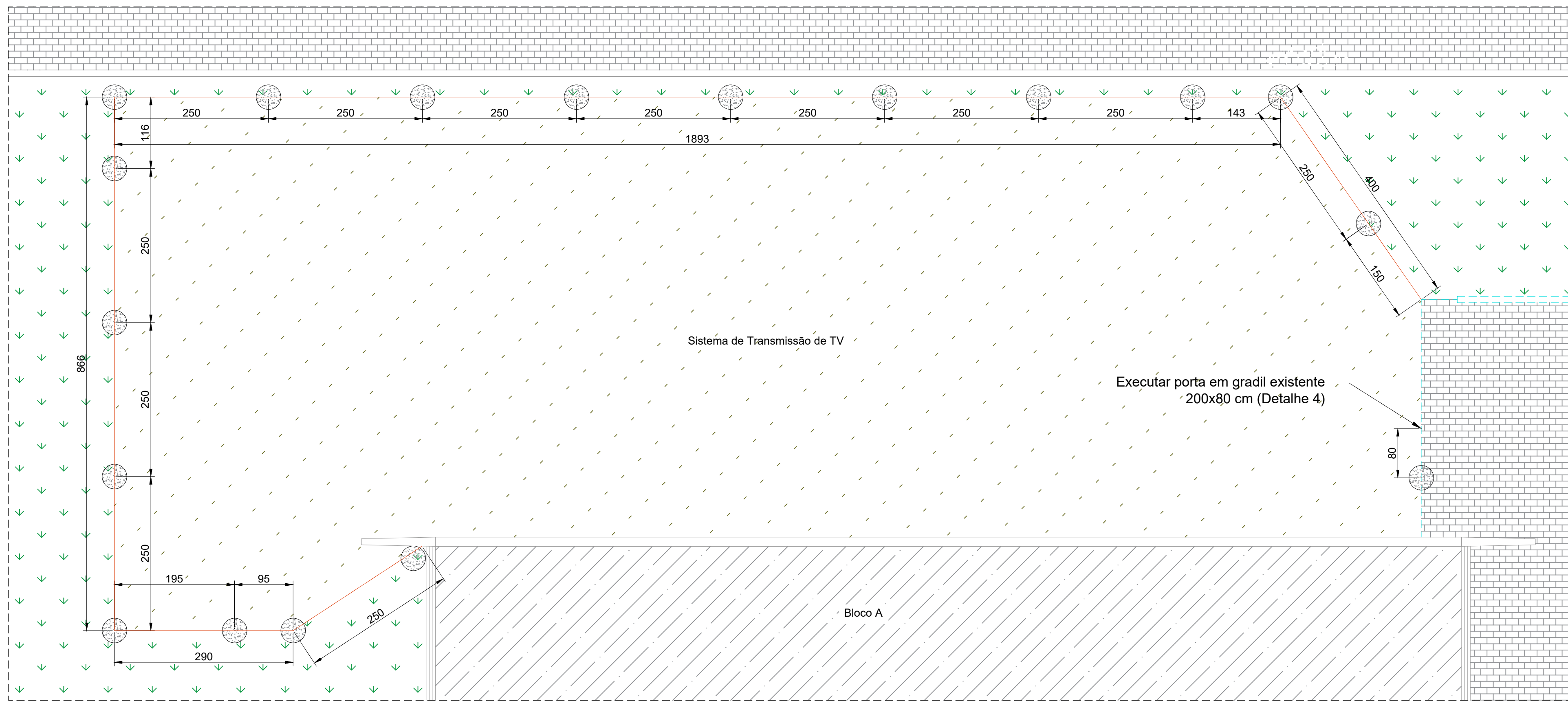
PLANTA BAIXA Cercamento das Antenas Escala 1:50
