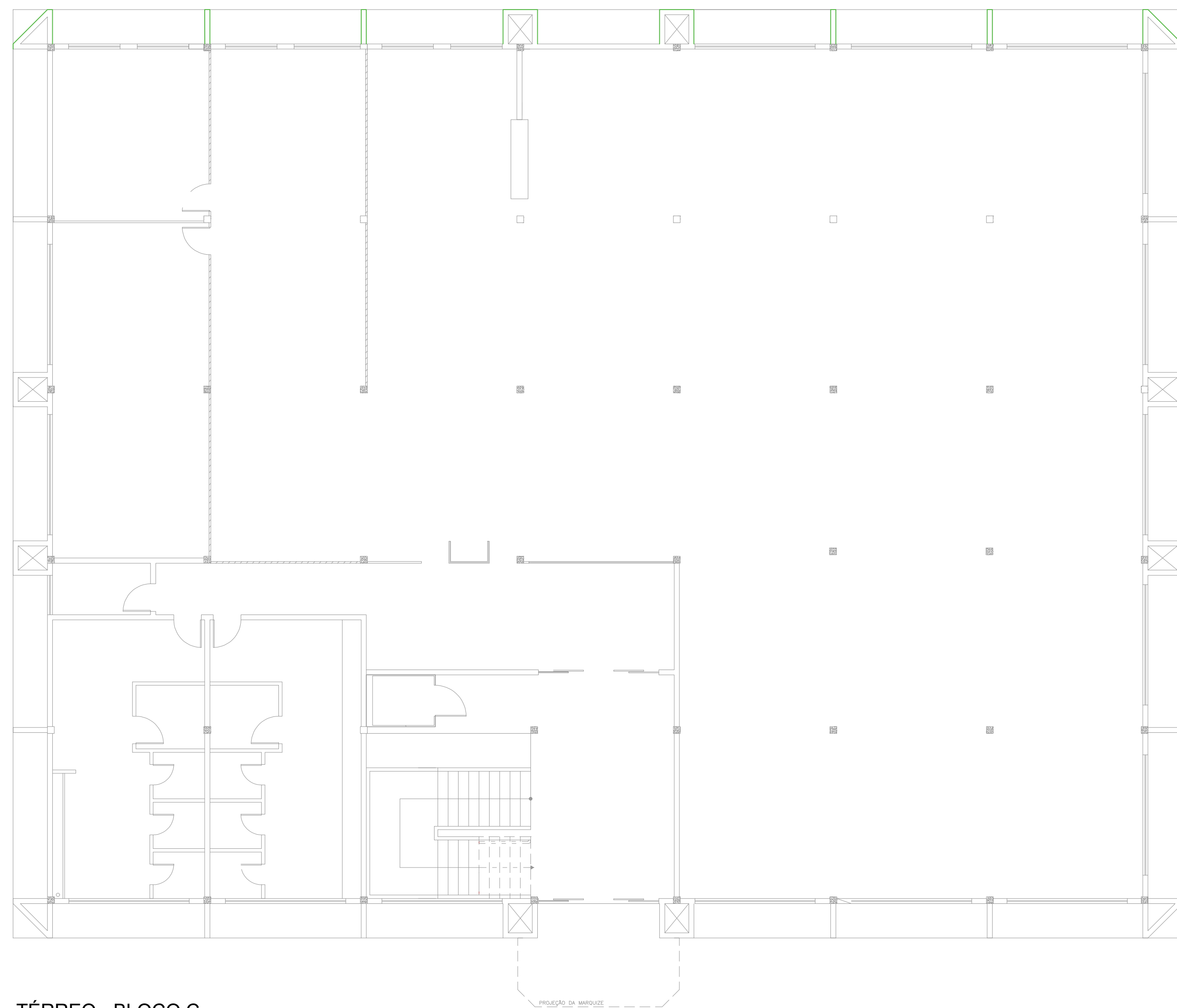
TÉRREO - BLOCO C Escala 1:100
