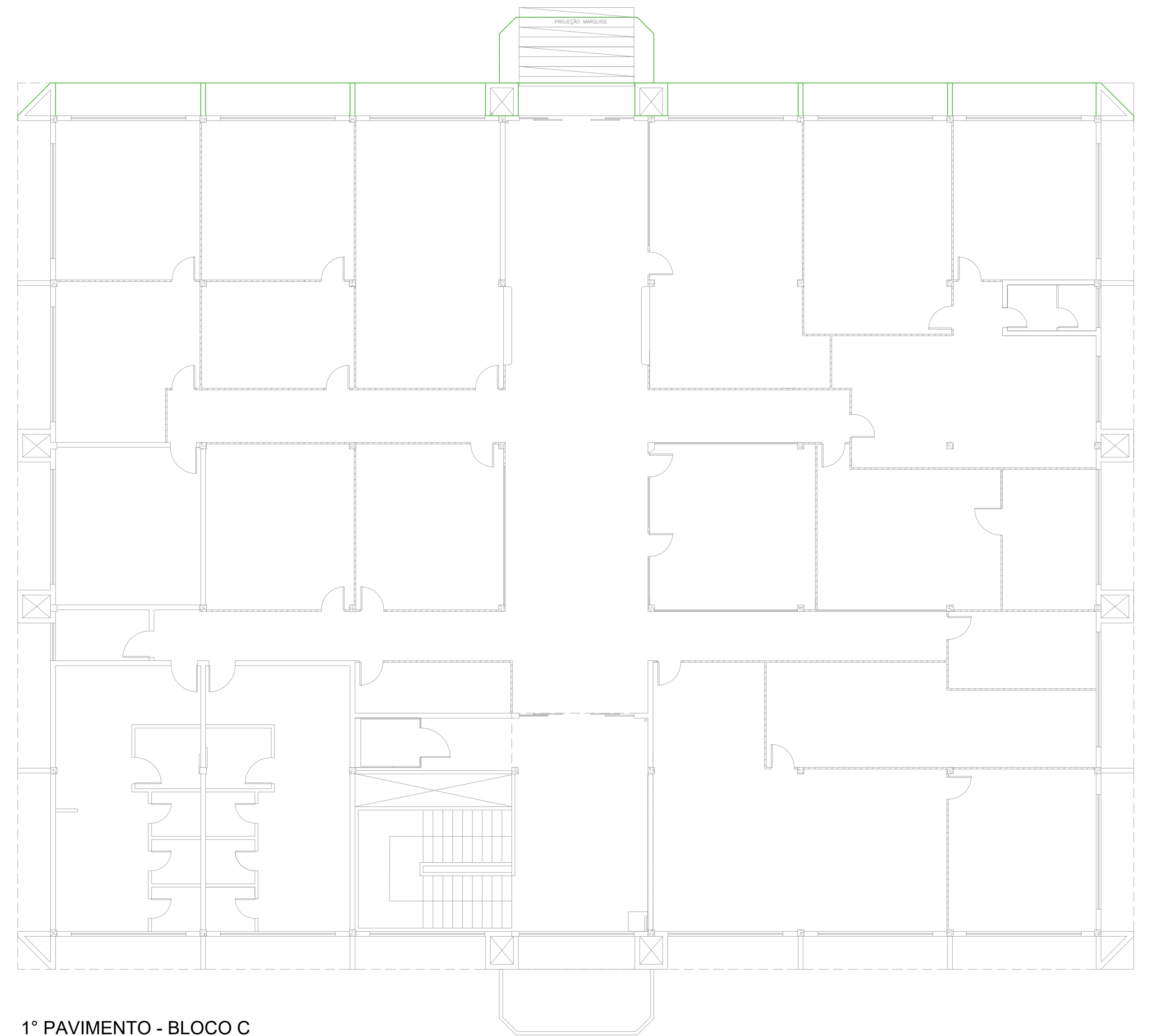
1º PAVIMENTO - BLOCO C Escala 1:100
