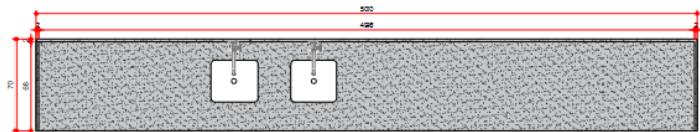
PLANTA TAMPO ESCALA 1/25
