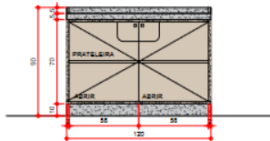
VISTA FRONTAL ESCALA 1/25
