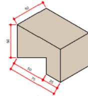
ISOMÉTRICA PUXADOR ESCALA 1/1
