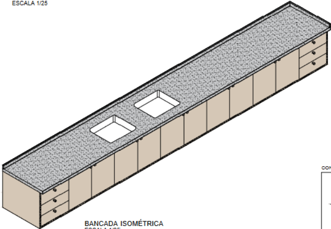
BANCADA ISOMÉTRICA ESCALA 1/25
