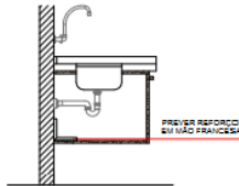
CORTE ESCALA 1/25
