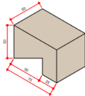
ISOMÉTRICA PUXADOR ESCALA 1/1
