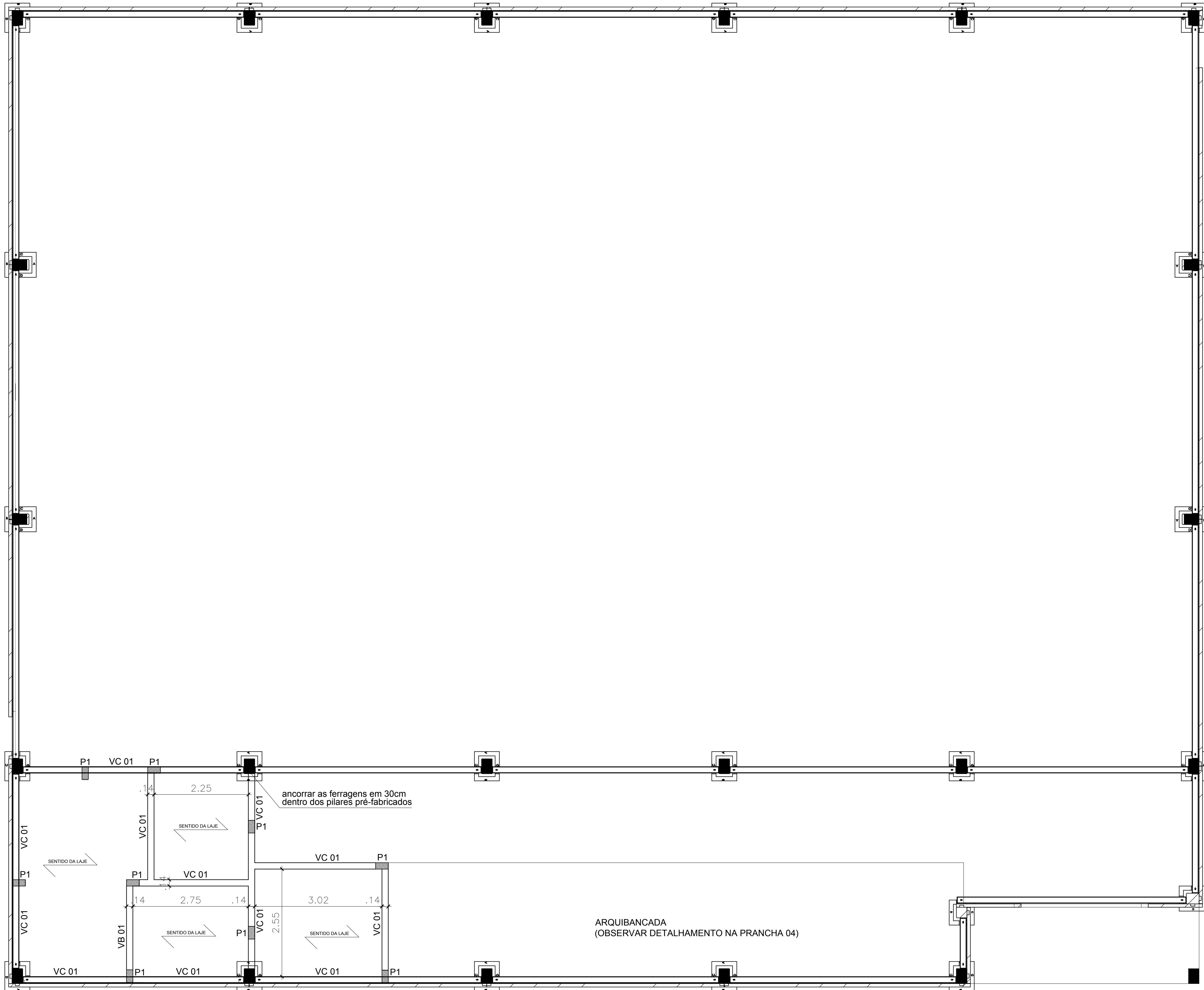
PLANTA BAIXA PILARES, VIGAS DE COBERTURA E LAJE ESCALA 50 / 100
