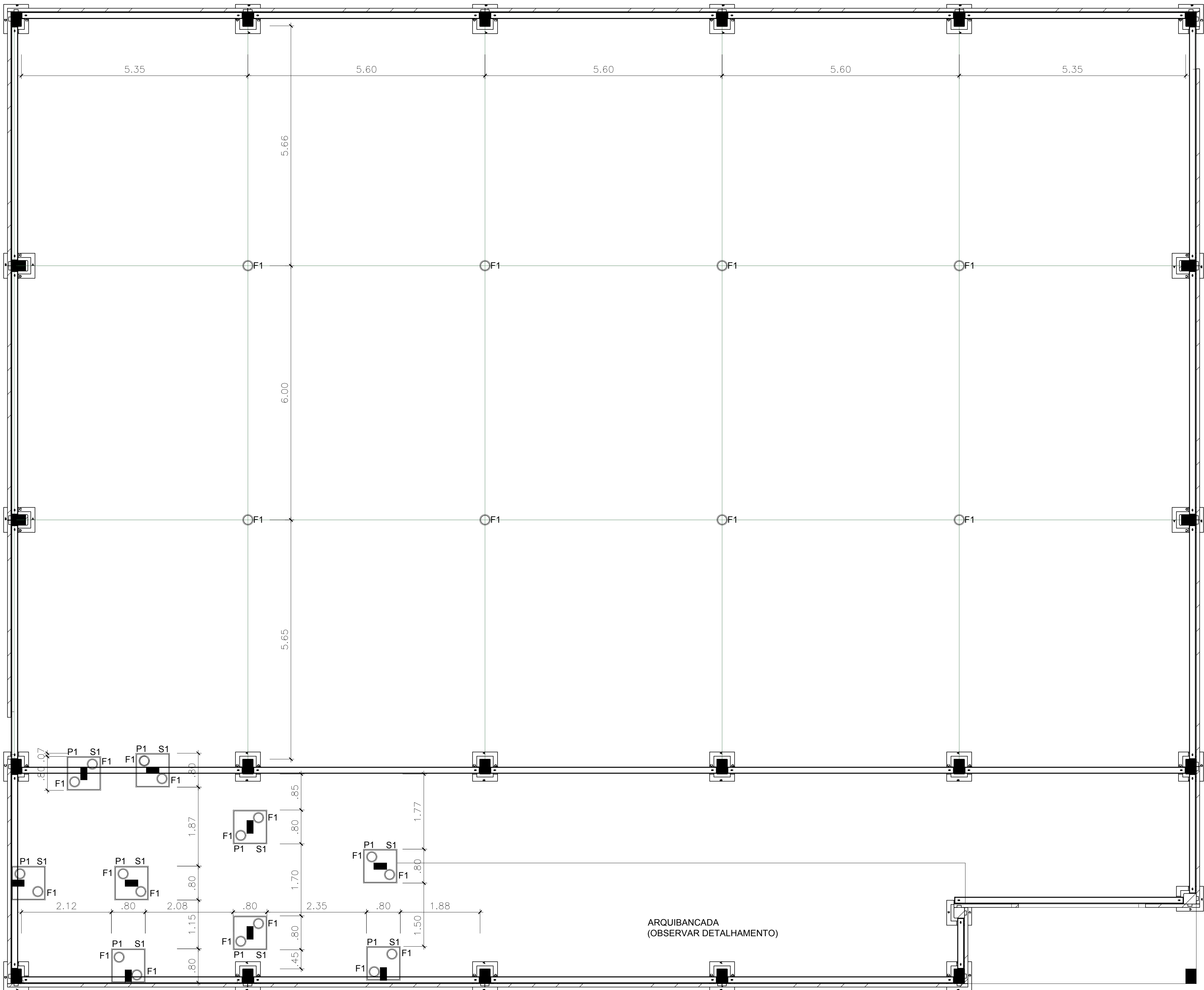
PLANTA BAIXA DA FUNDAÇÃO ESCALA 50 / 100
