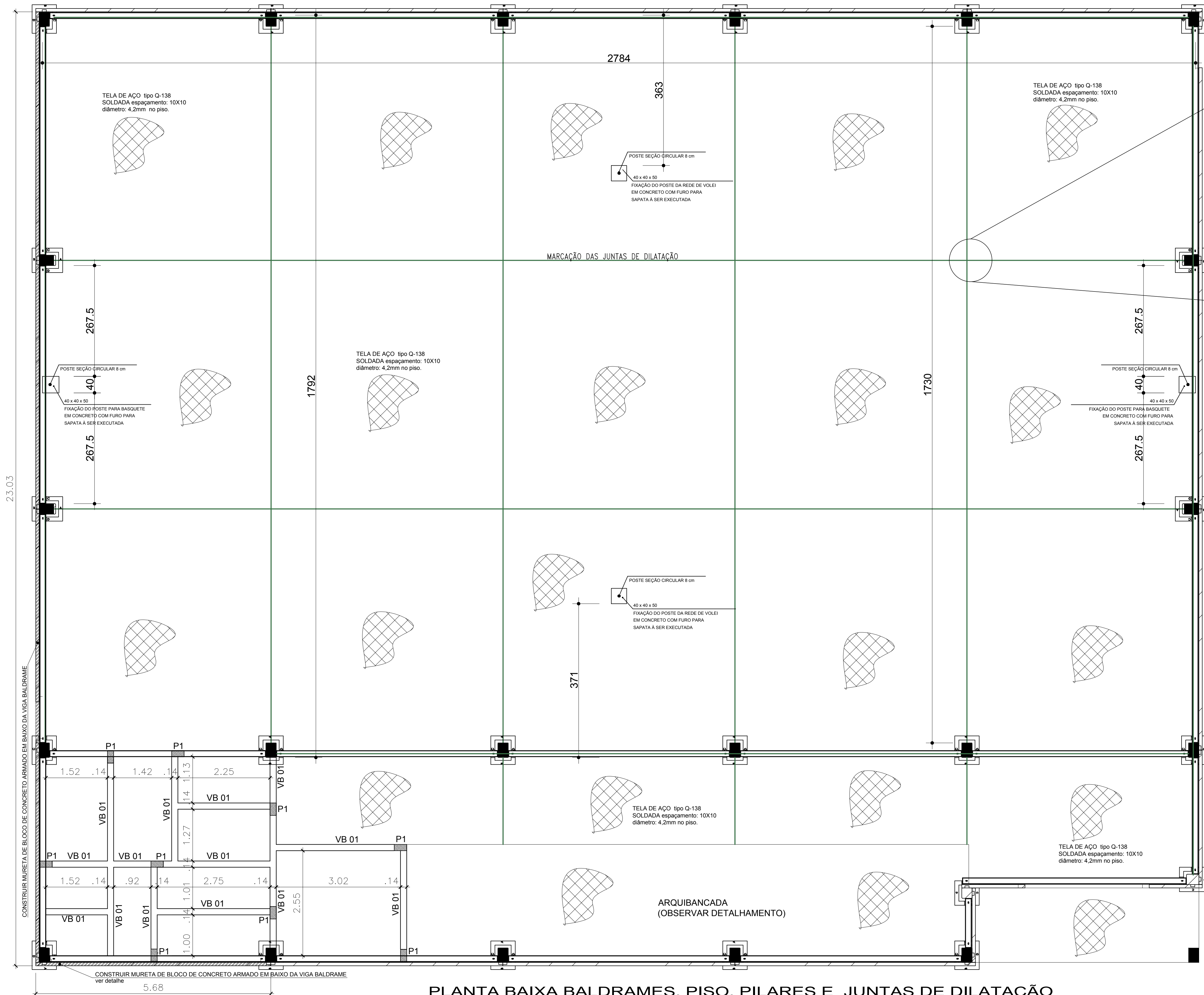
PLANTA BAIXA BALDRAMES, PISO, PILARES E JUNTAS DE DILATAÇÃO ESCALA 50 / 100
