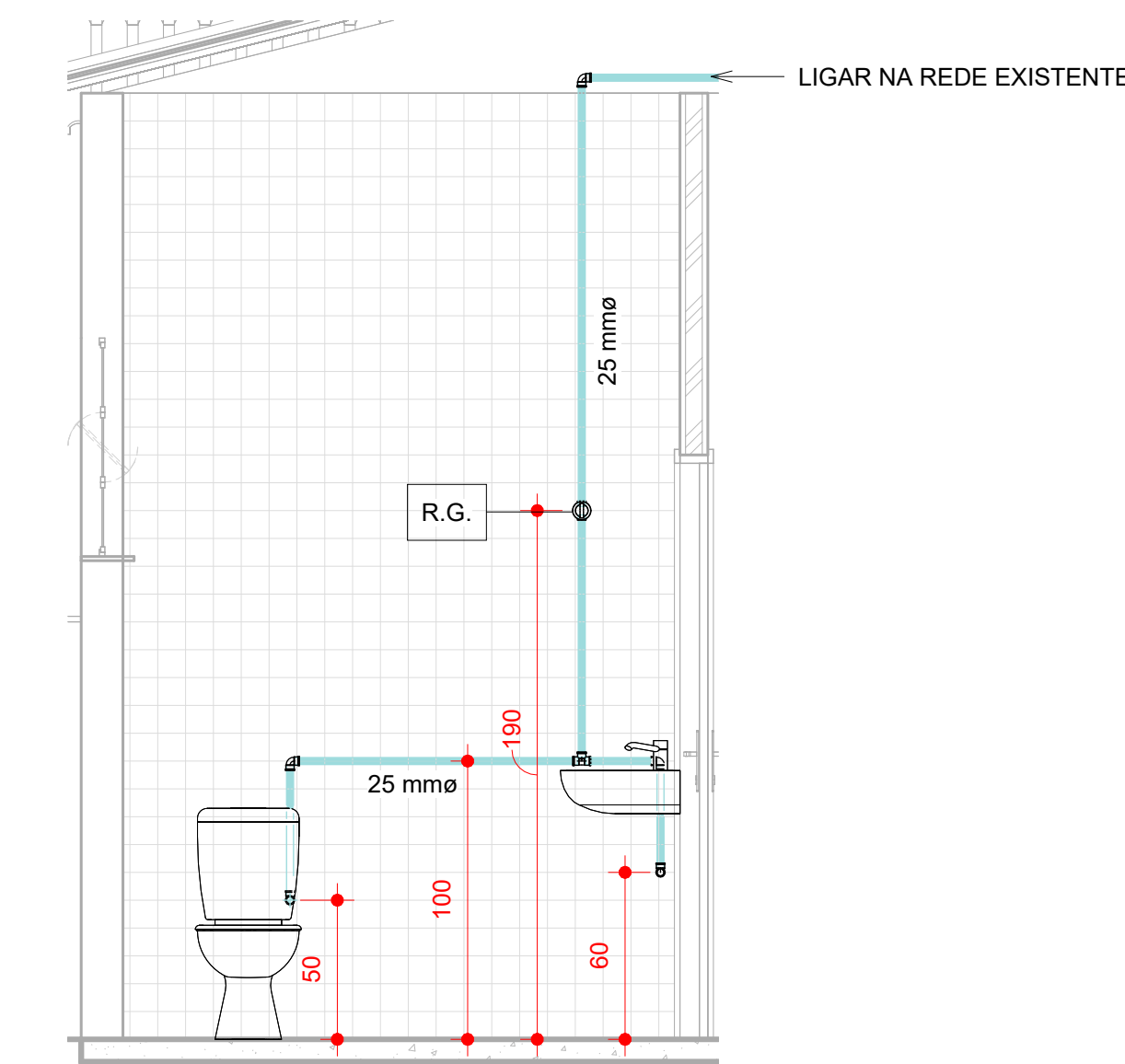
3 D.I.A 01 1 : 25
