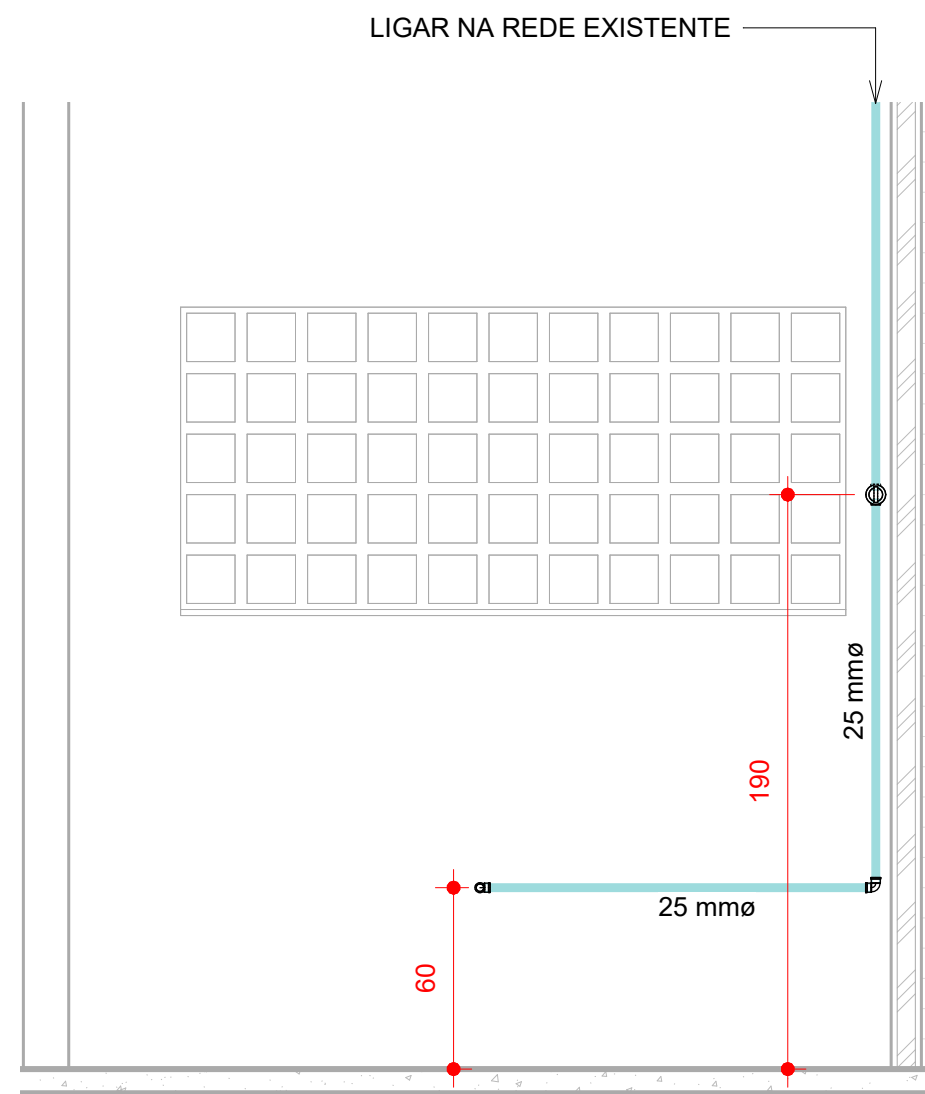
5 D.I.A 02 1 : 25
