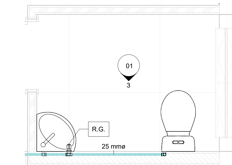
2 D.I.A 01 1 : 20
