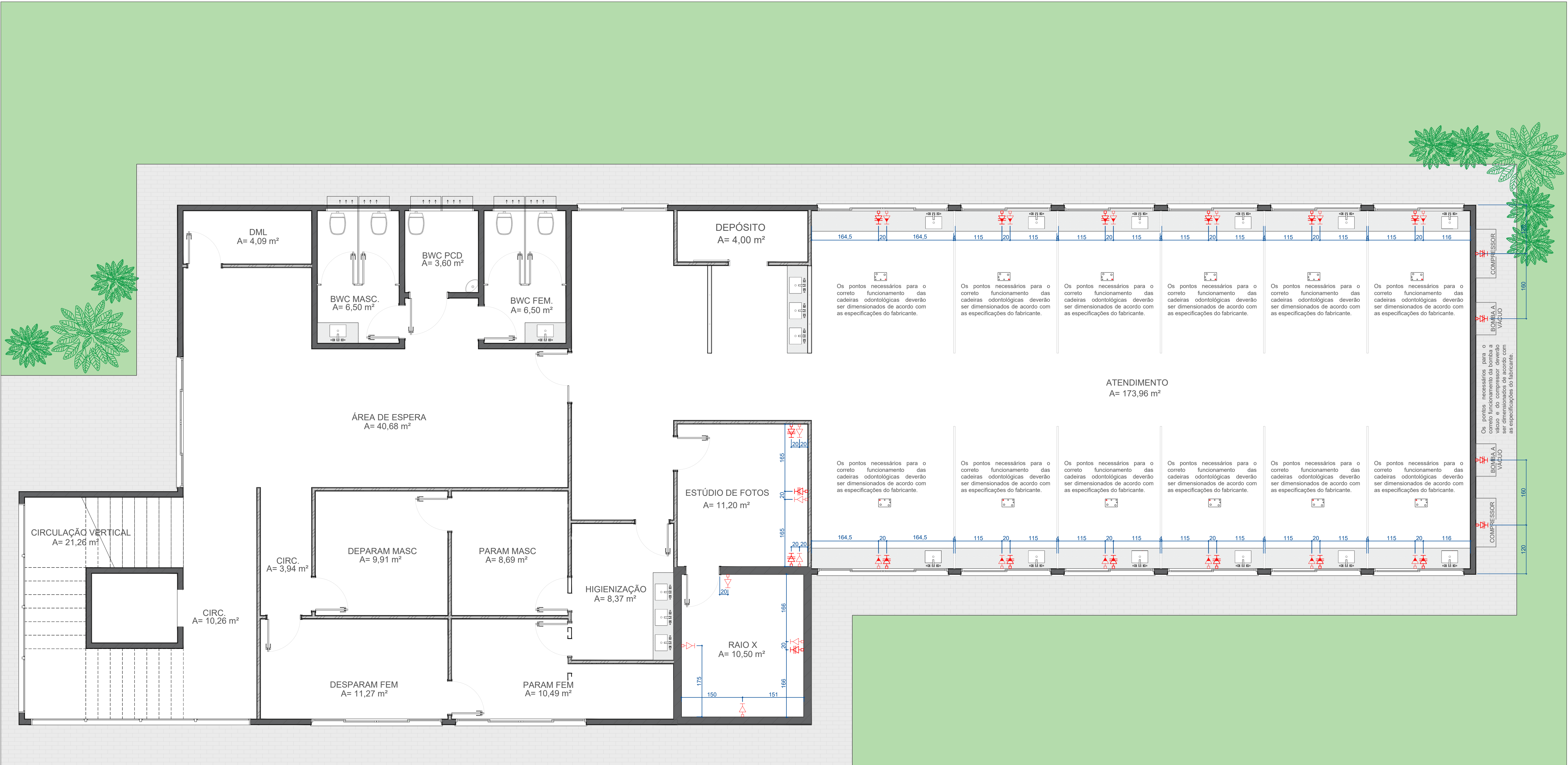
PLANTA BAIXA - Térreo Pontos Elétricos Esc:.....1/50
