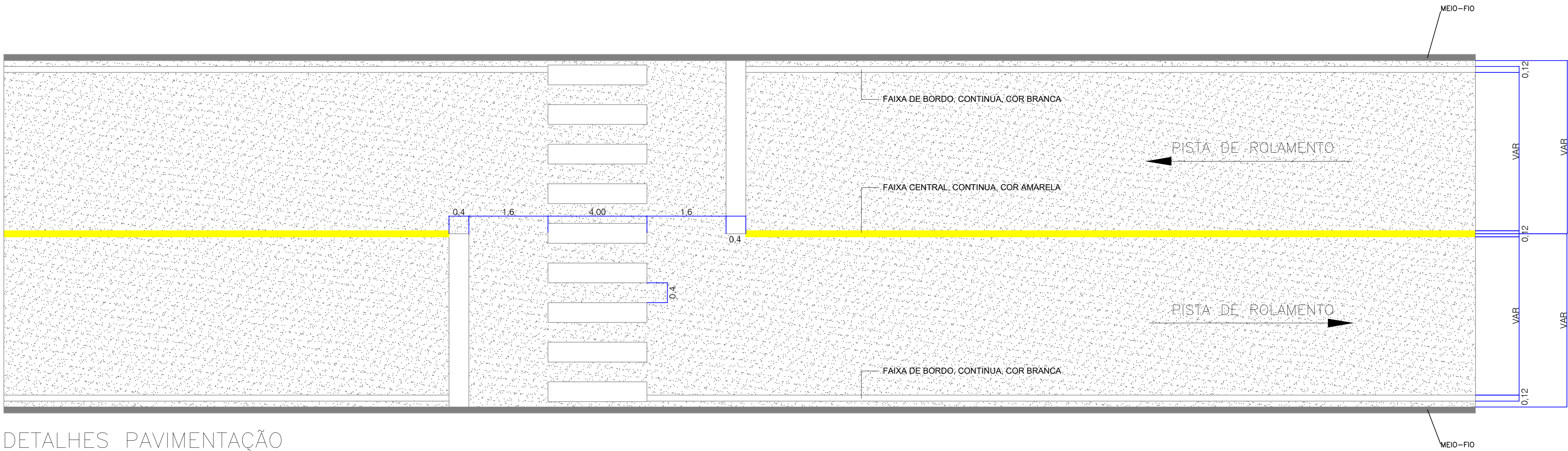
DETALHES PAVIMENTAÇÃO
