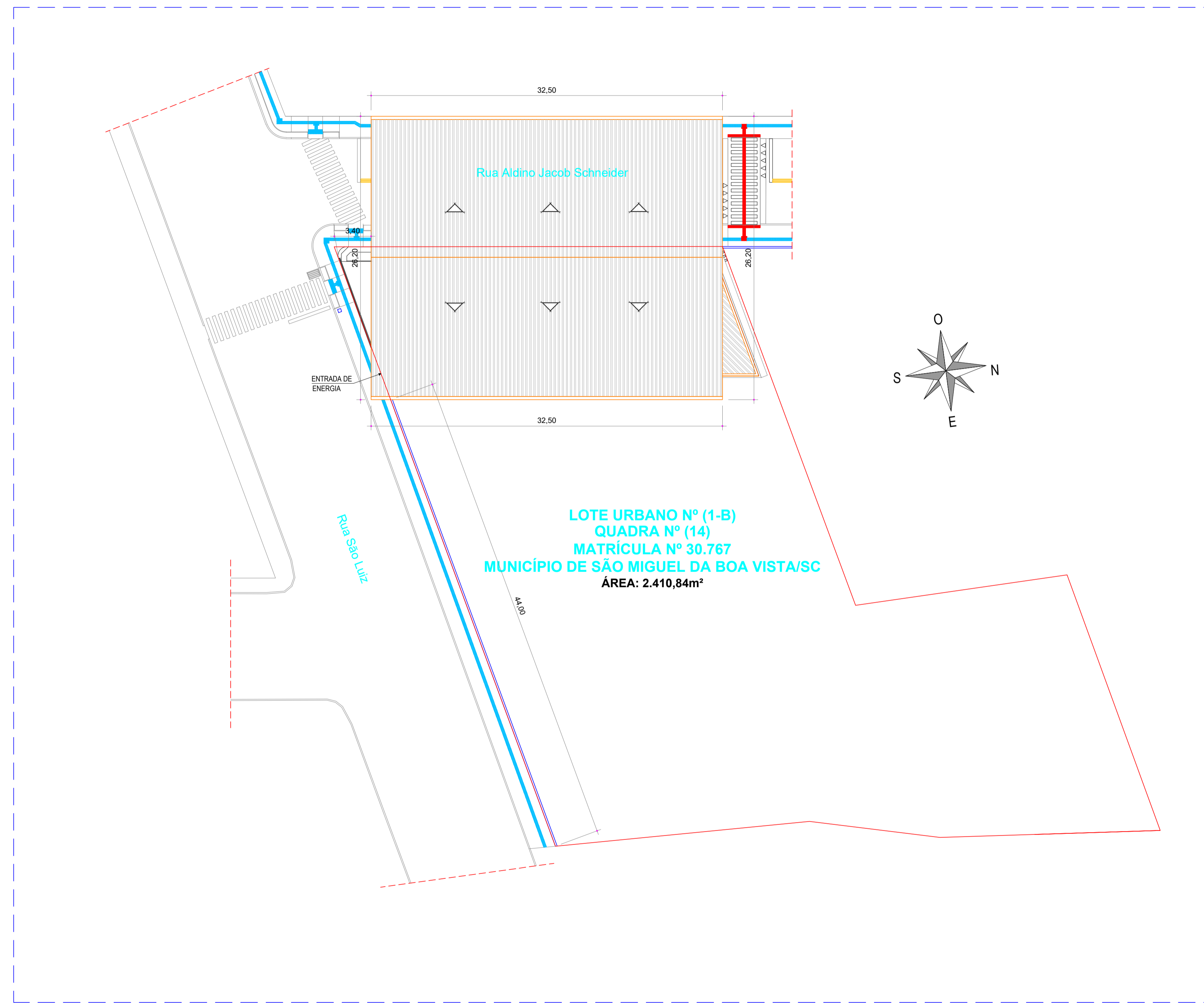
Planta de Implantação Escala= 1 : 250
