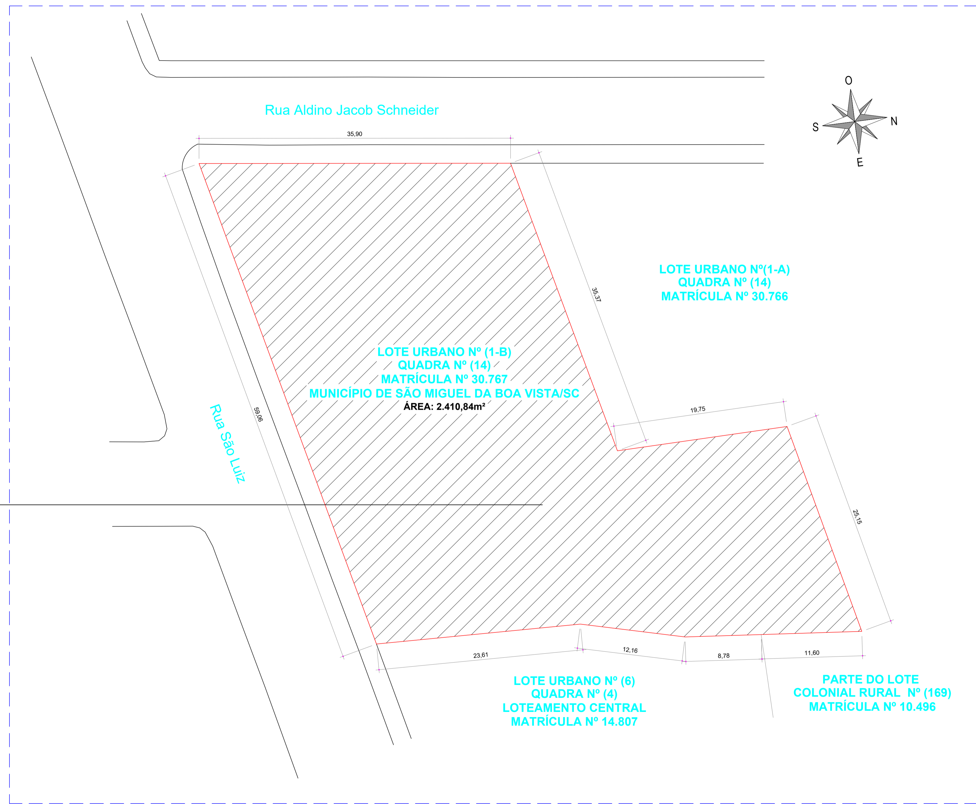
Planta de Situação Escala= 1 : 250
