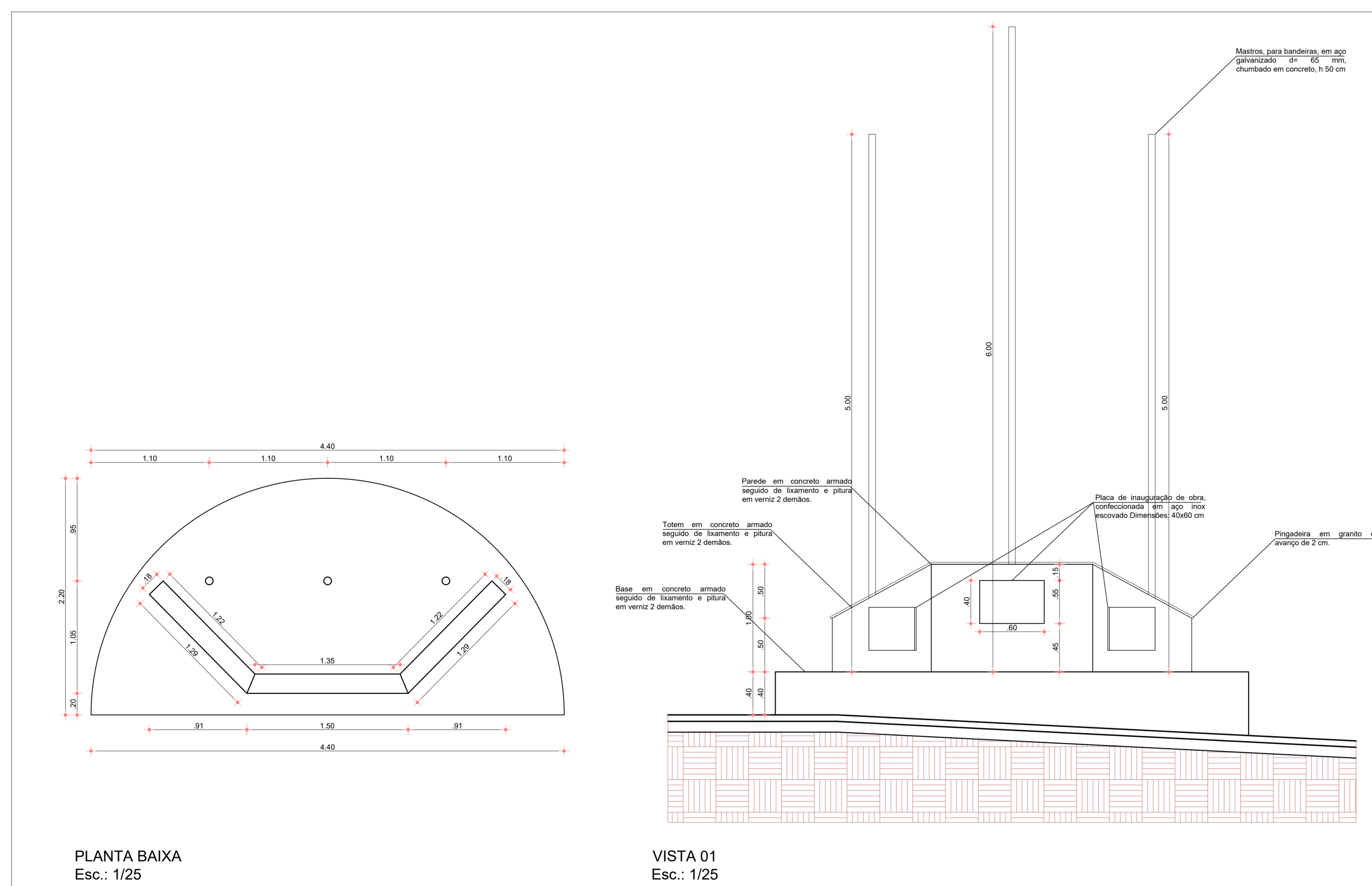
DETALHE DO TOTEM COMEMORATIVO
