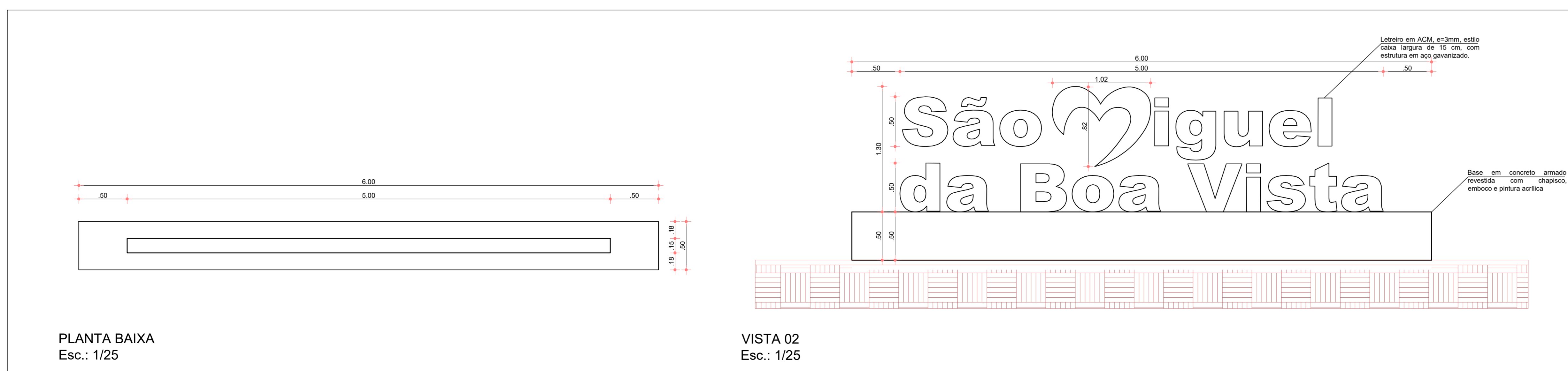
DETALHE DO LETREIRO EM ACM
