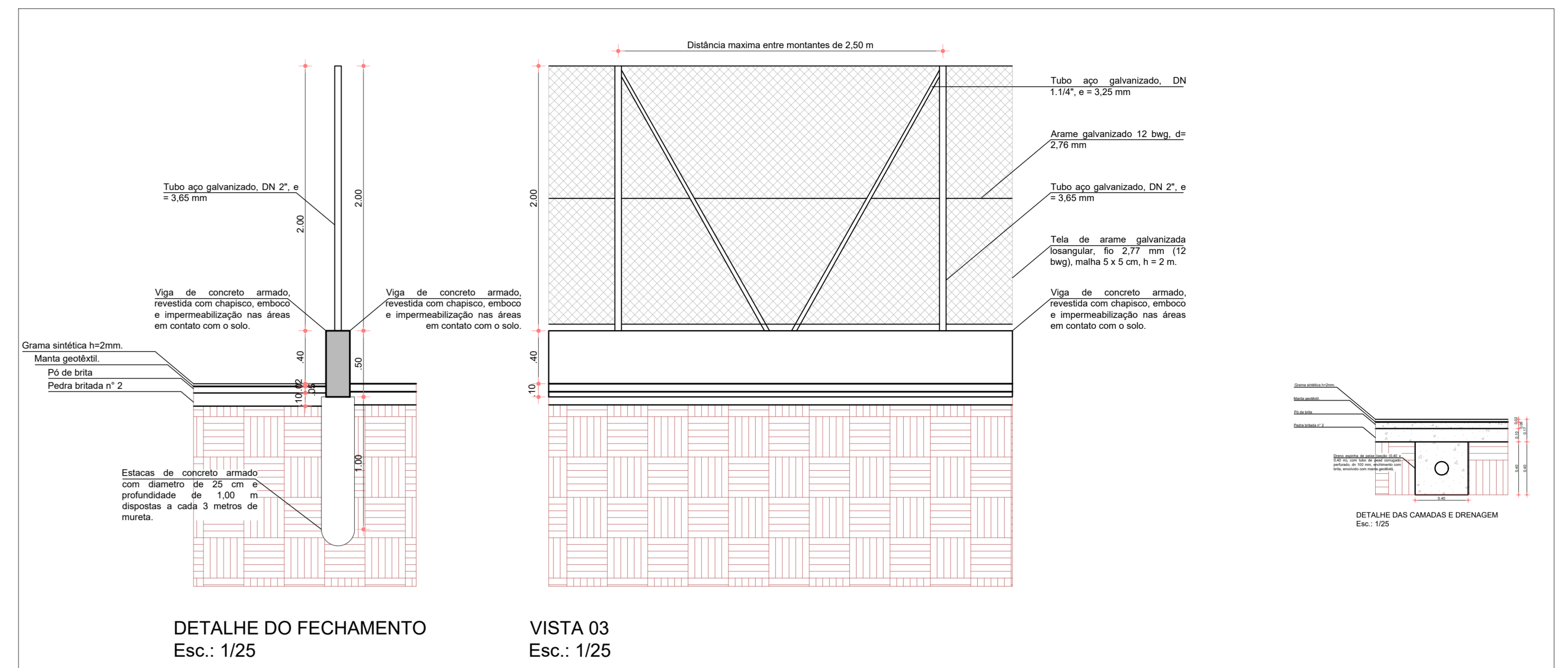
DETALHES DO PLAYGROUD
