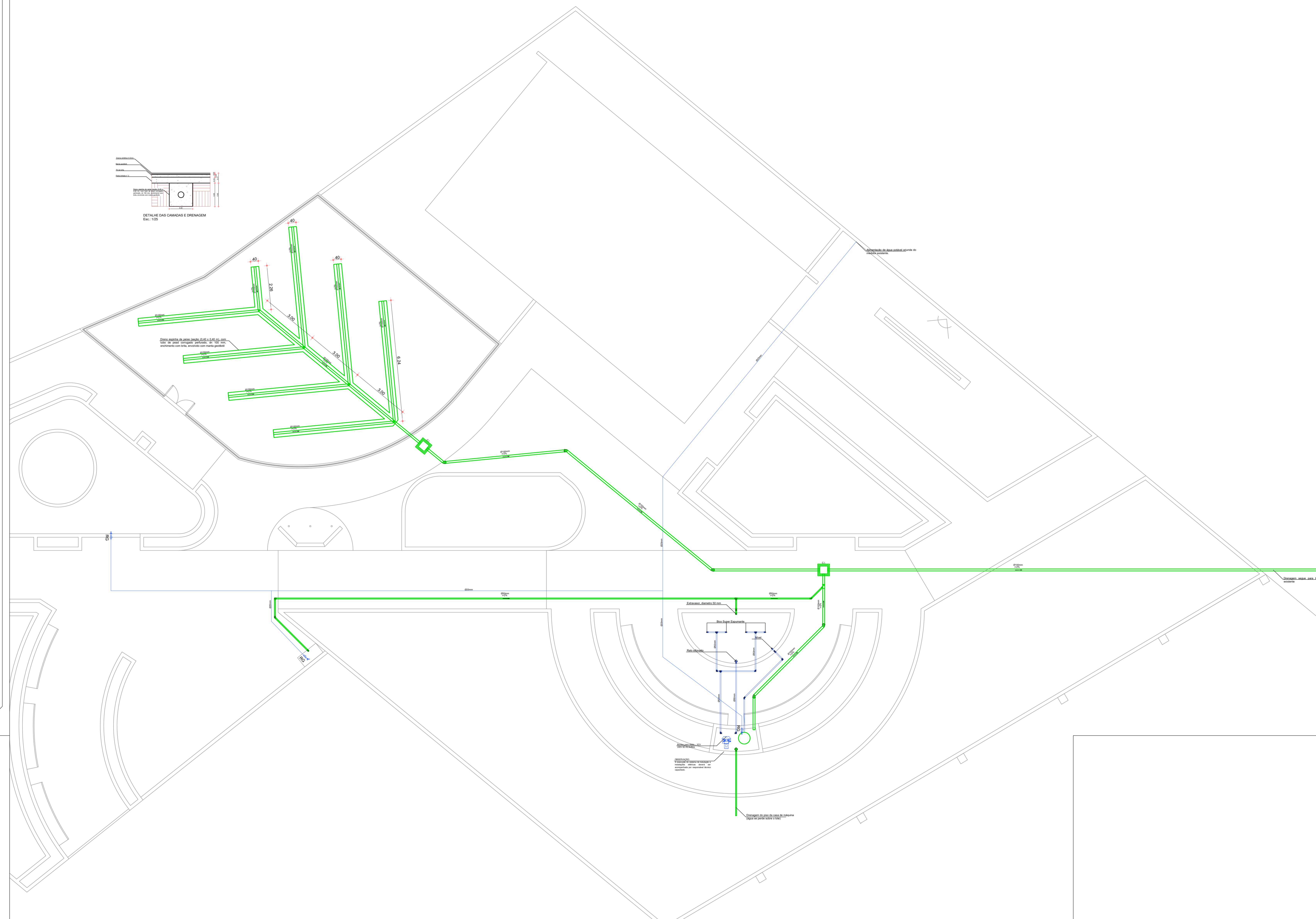
PLANTA BAIXA - Hidráulico e Drenagem Esc.: 1/75
