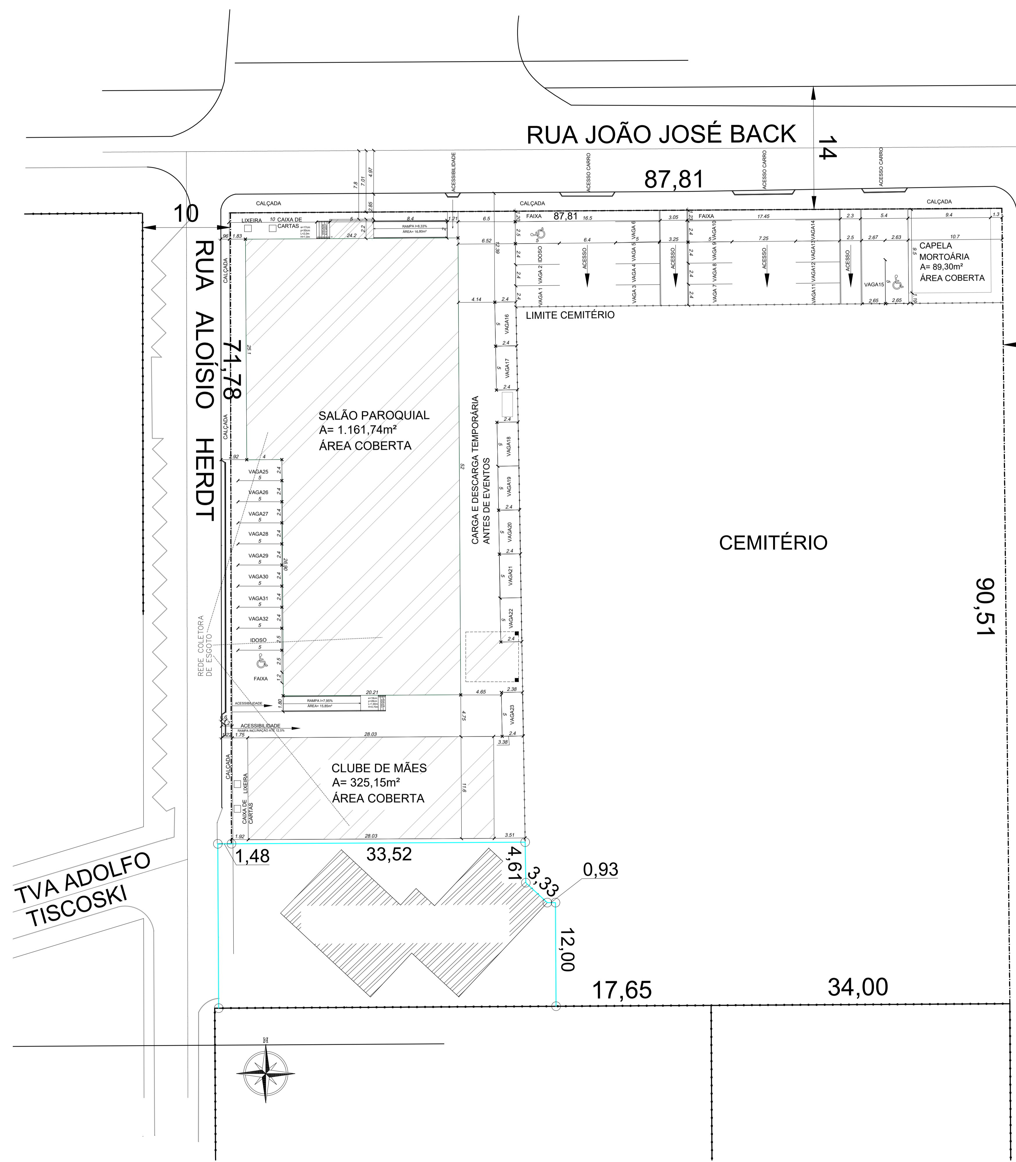
11 PLANTA DE LOCAÇÃO E SITUAÇÃO ESCALA: 1/250
