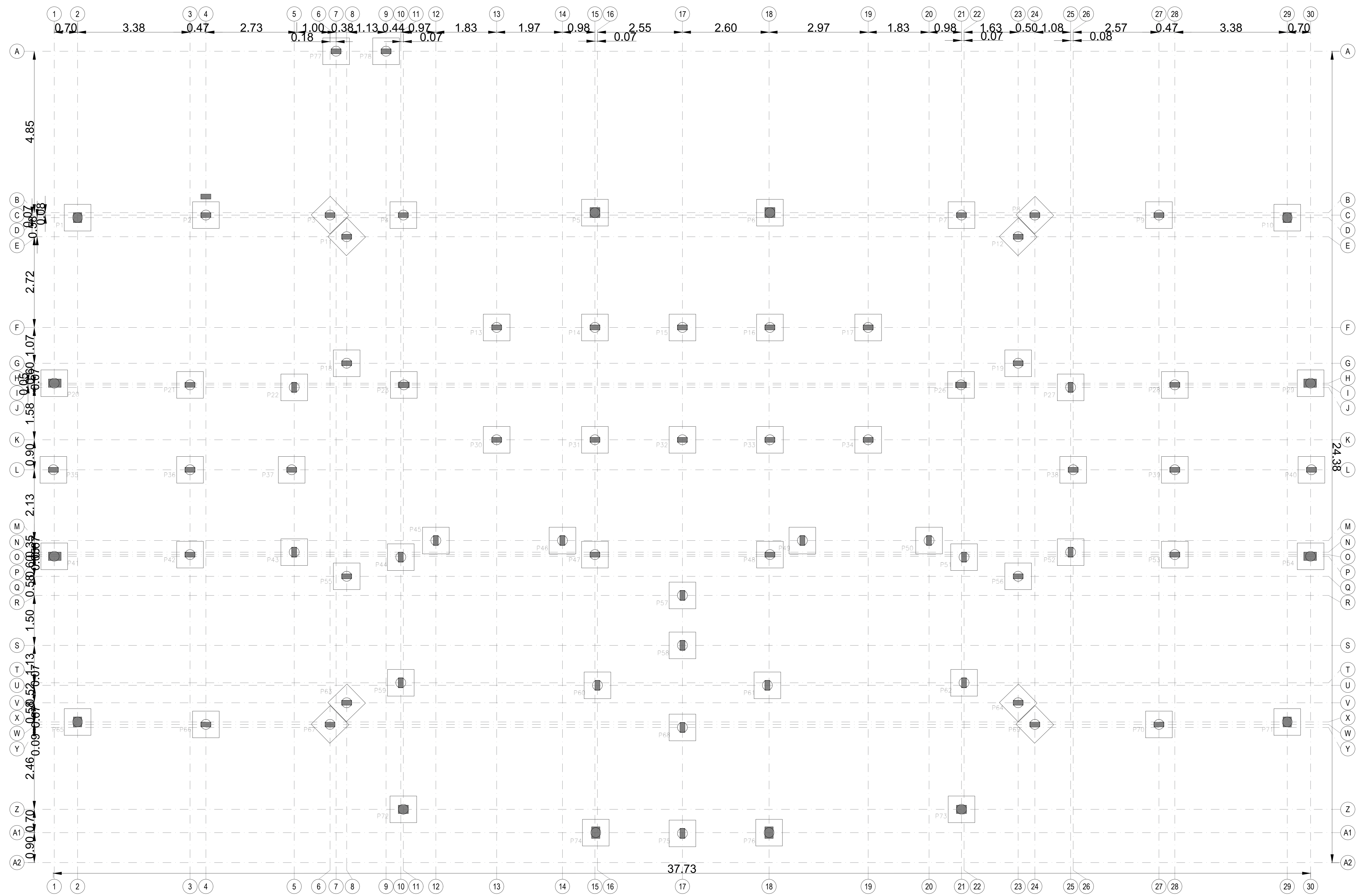
LOCAÇÃO DE BLOCOS DE COROAMENTO Escala: 1/100
