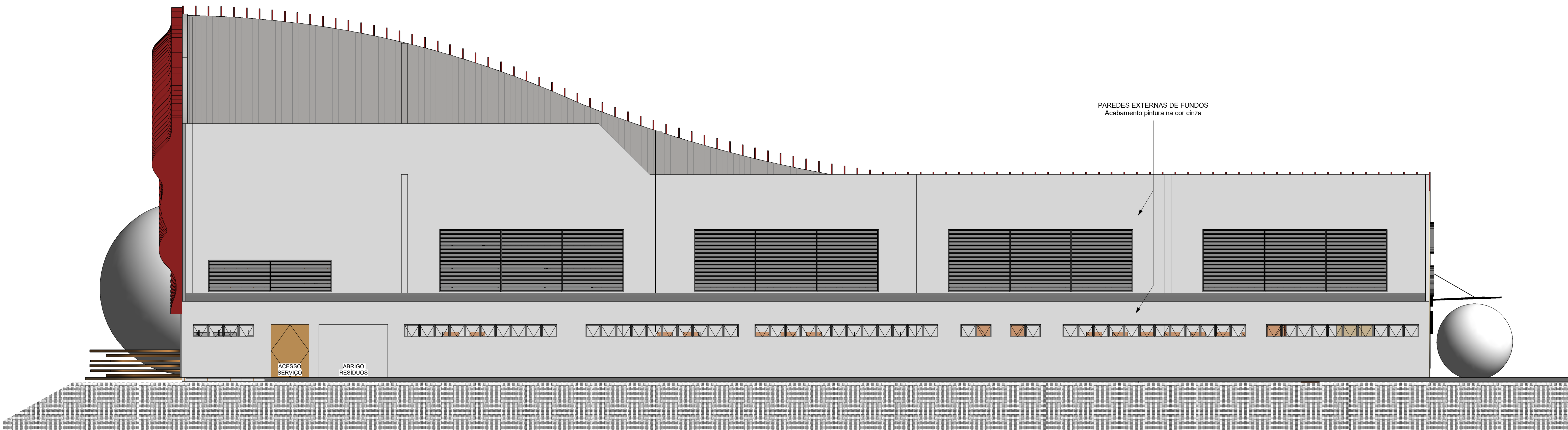
4 Elevação Posterior 1 : 75
