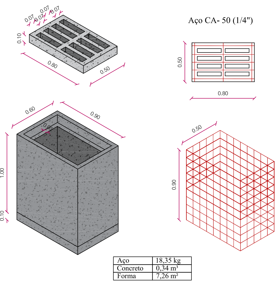
Detalhes boca de lobo e grelha Esc: 1:25
