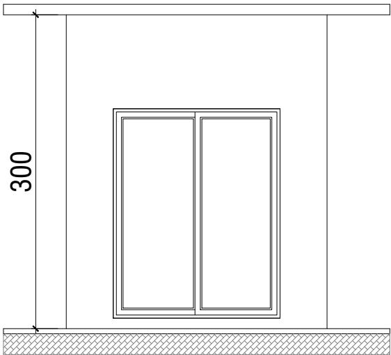
FACHADA FRONTAL ESC. 1/50
