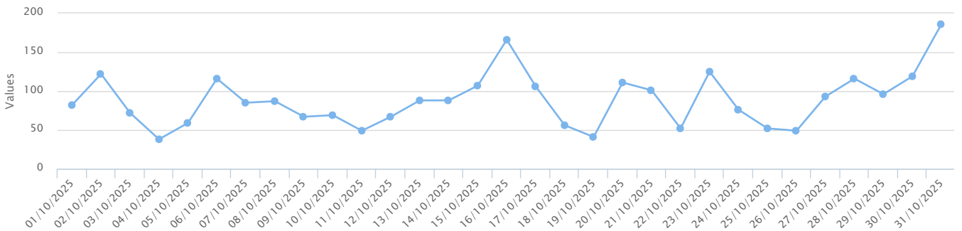
Unique Browsers
