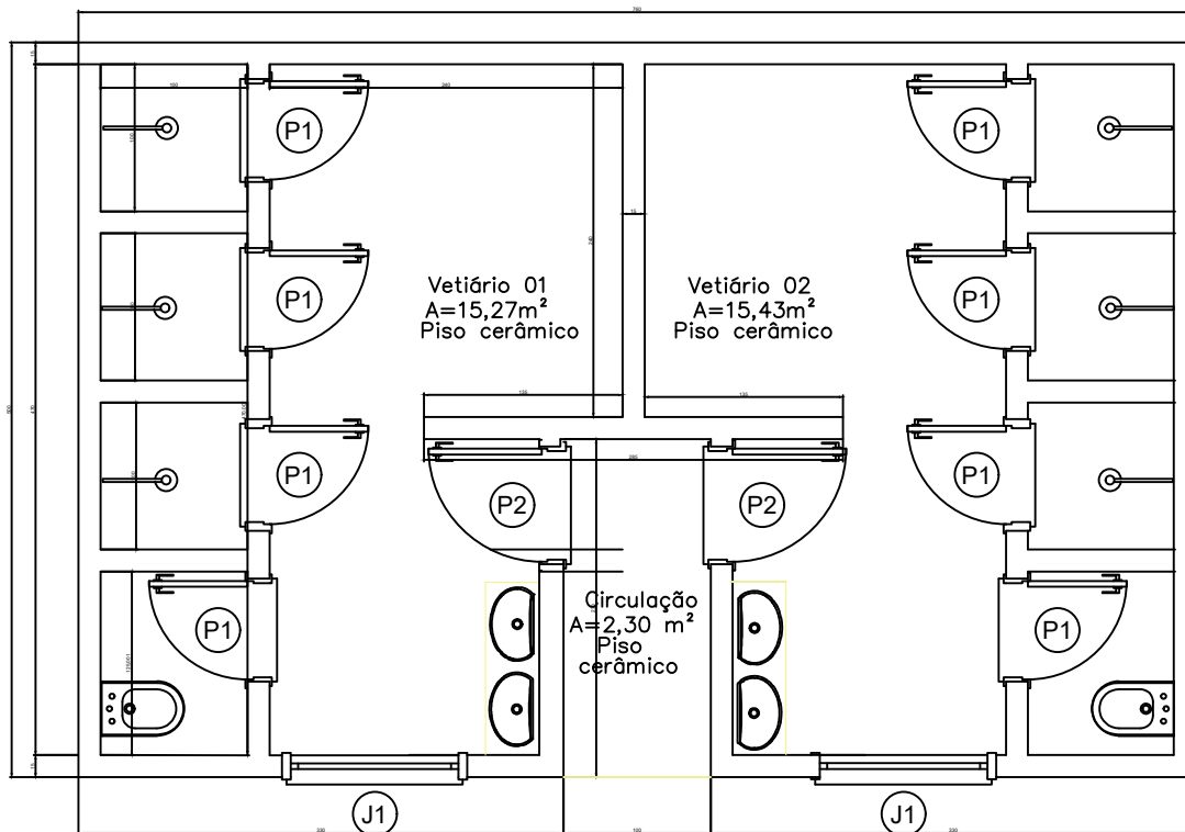
01 PLANTA BAIXA A:38,00 m 2 Escala 1:100
