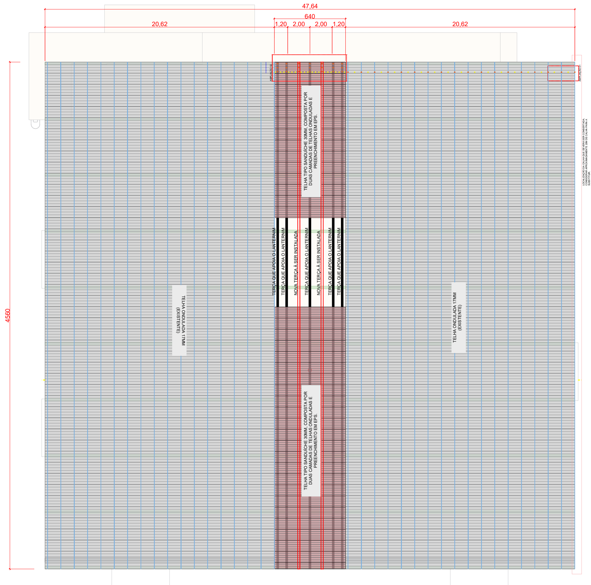
Planta de Cobertura reforma do lanternim ESCALA 1/200
