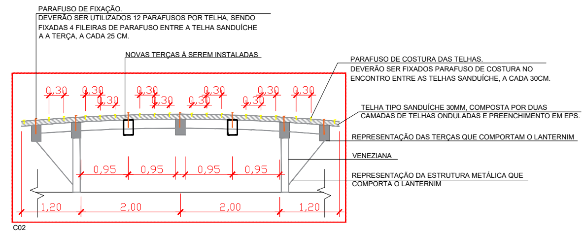
AMPLIAÇÃO 01 PADRÃO DOS PARAFUSOS DE COSTURA E DE FIXAÇÃO DA COBERTURA TOTAL DO TELHADO.
