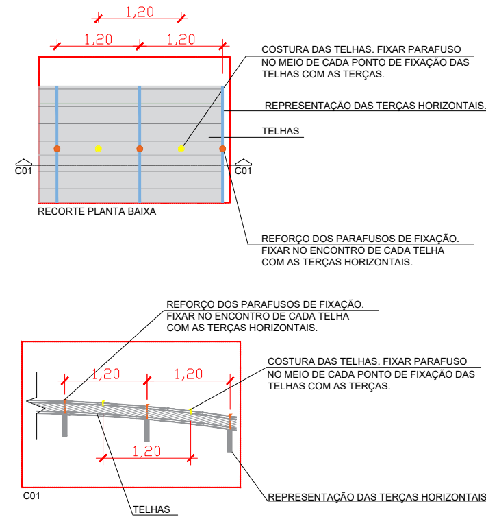
AMPLIAÇÃO 01 PADRÃO DOS PARAFUSOS DE COSTURA E DE FIXAÇÃO DA COBERTURA TOTAL DO TELHADO.
