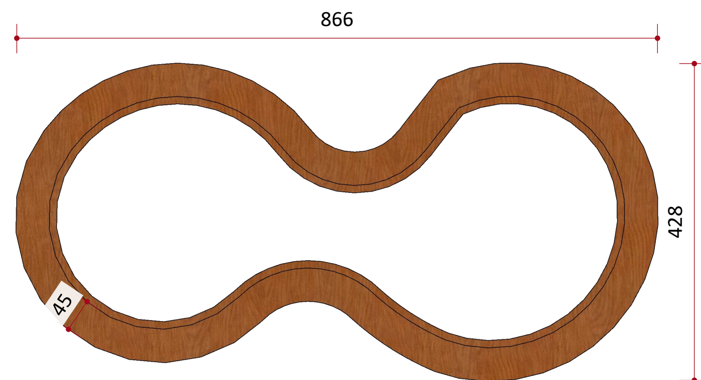
4 PLANTA BAIXA BANCO SEM ESCALA
