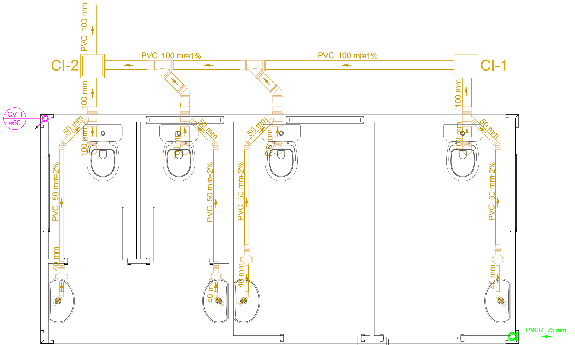
PLANTA BAIXA SANITÁRIO
