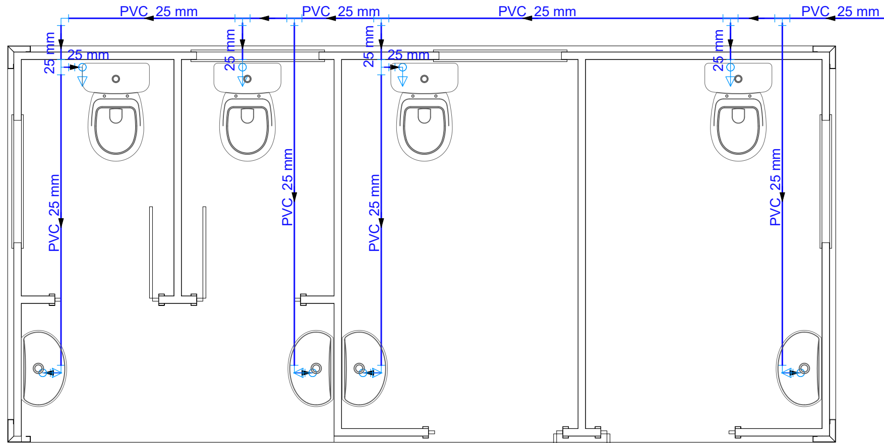
PLANTA BAIXA HIDRAULICO
