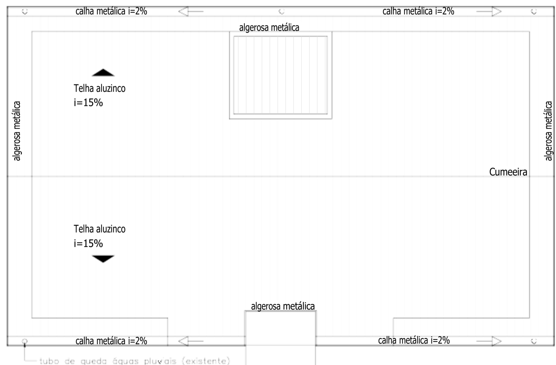
PLANTA DE COBERTURA Escala 1:50
