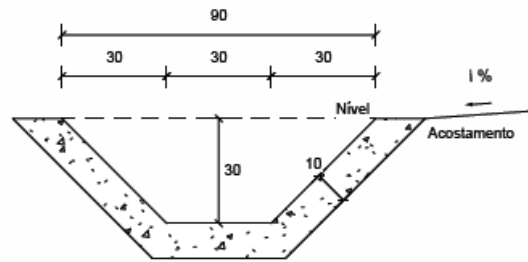
Seção transversal
