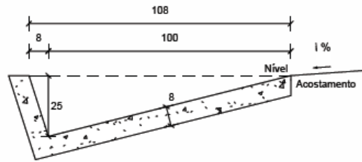
Seção transversal
