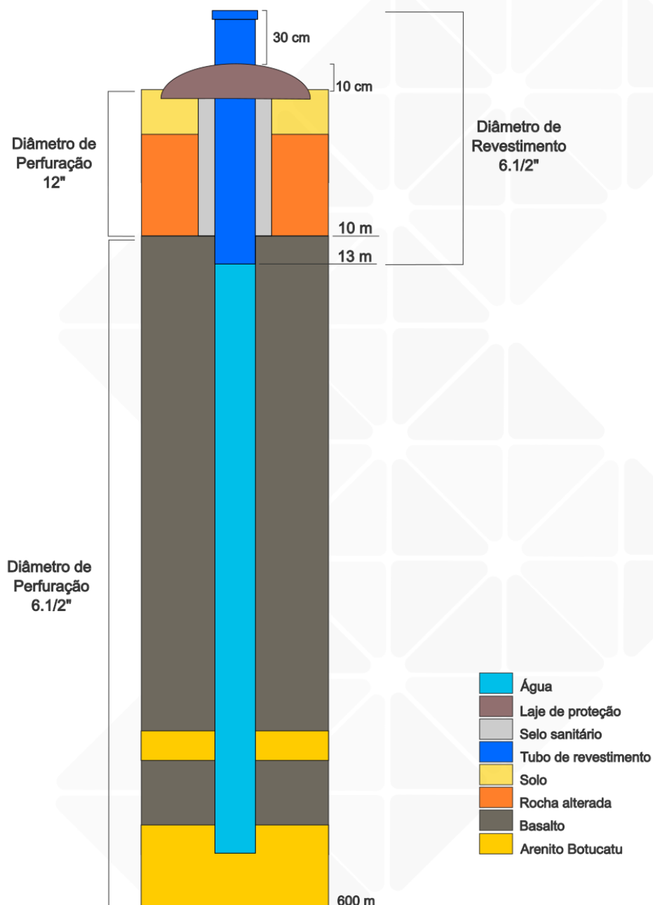
Figura 3: Perfil geológico e construtivo do poço
