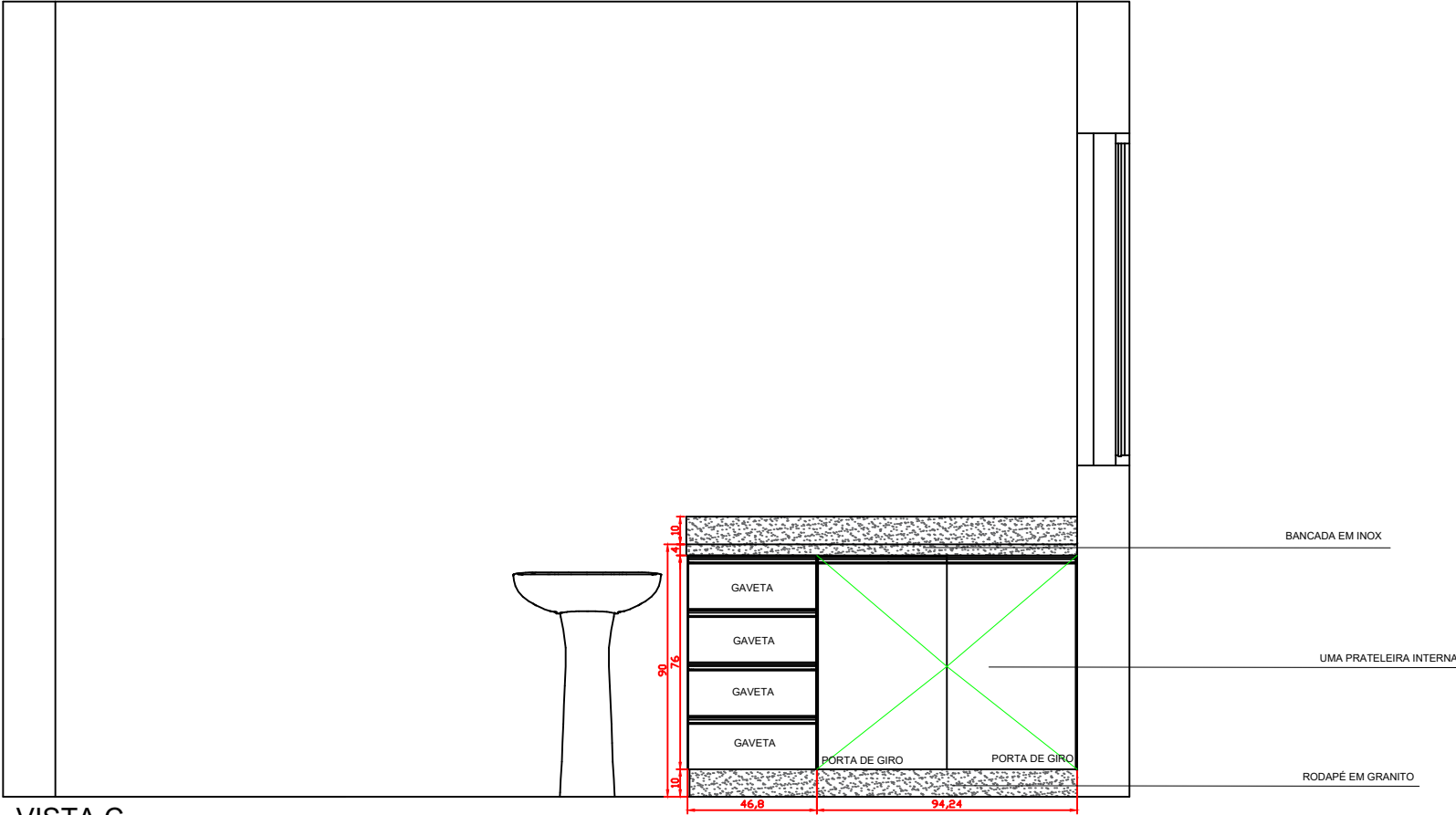
VISTA C 1:25
