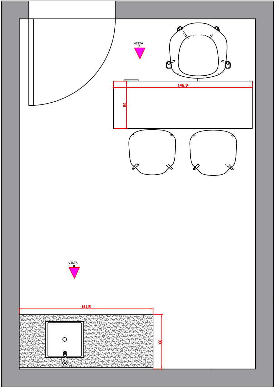
Planta Baixa Sala de Triagem 1:25
