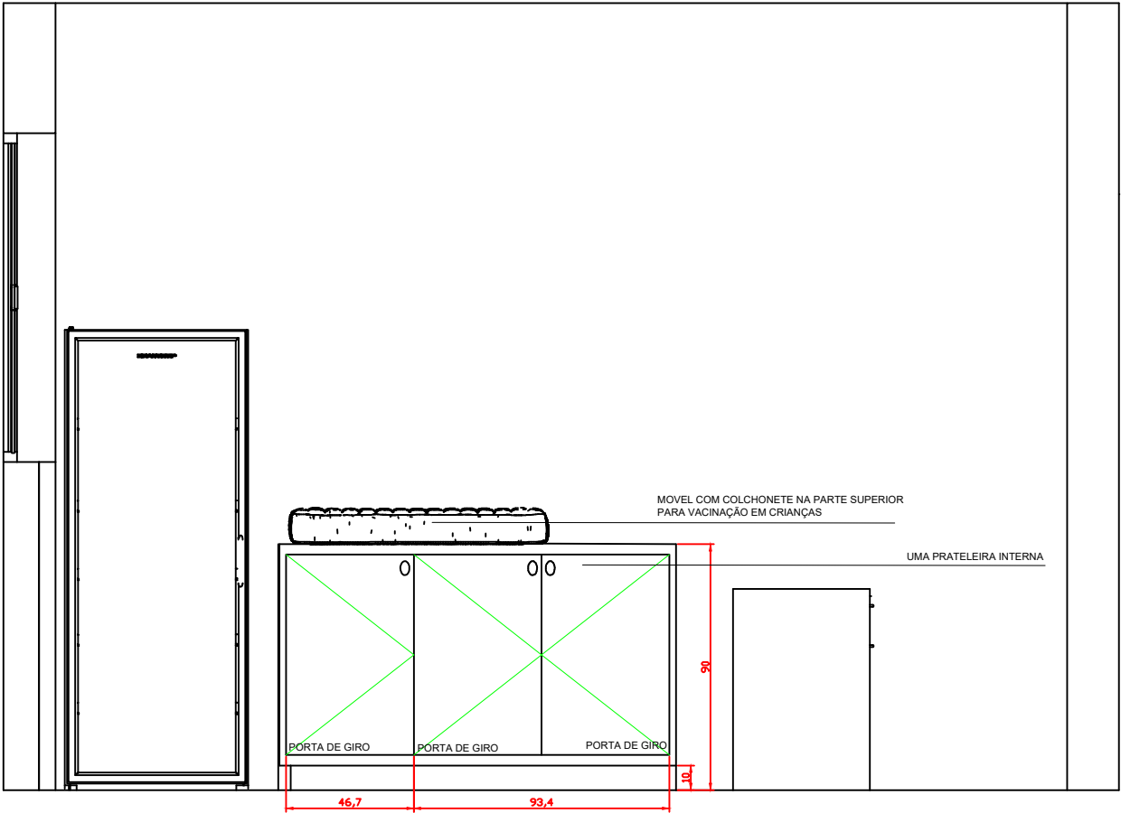
VISTA B 1:25
