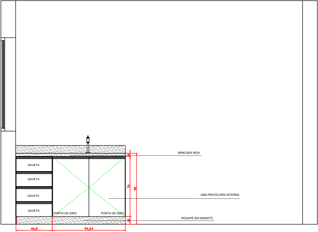
VISTA C 1:25
