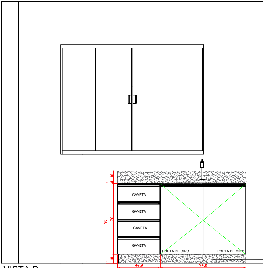
VISTA B 1:25
