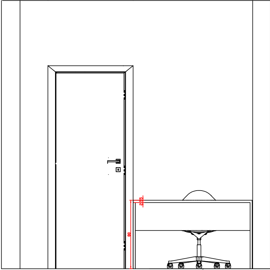
VISTA B 1:25
