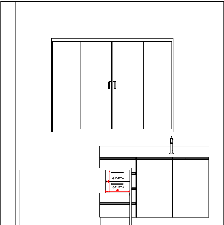
VISTA A 1:25
