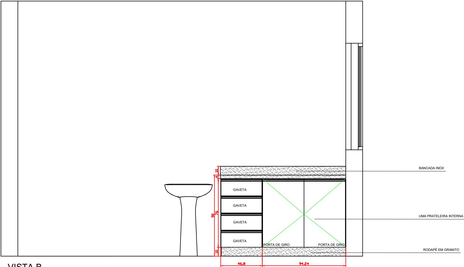
VISTA B 1:25
