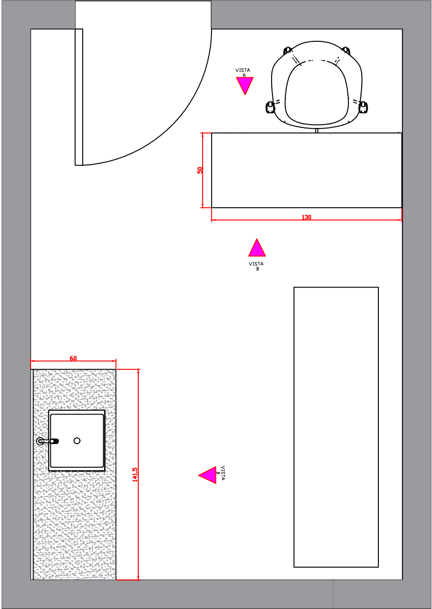
Planta Baixa Sala de Medicação 1:25
