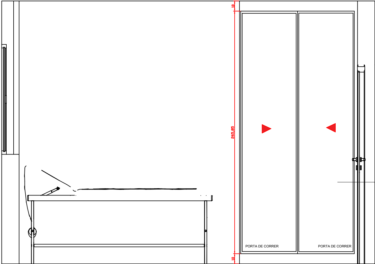
VISTA A 1:25
