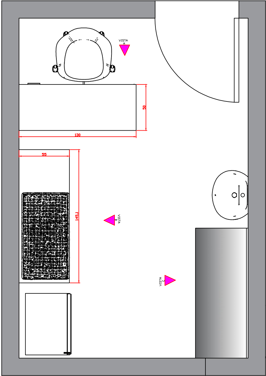
Planta Baixa Sala de Vacinas 1:25
