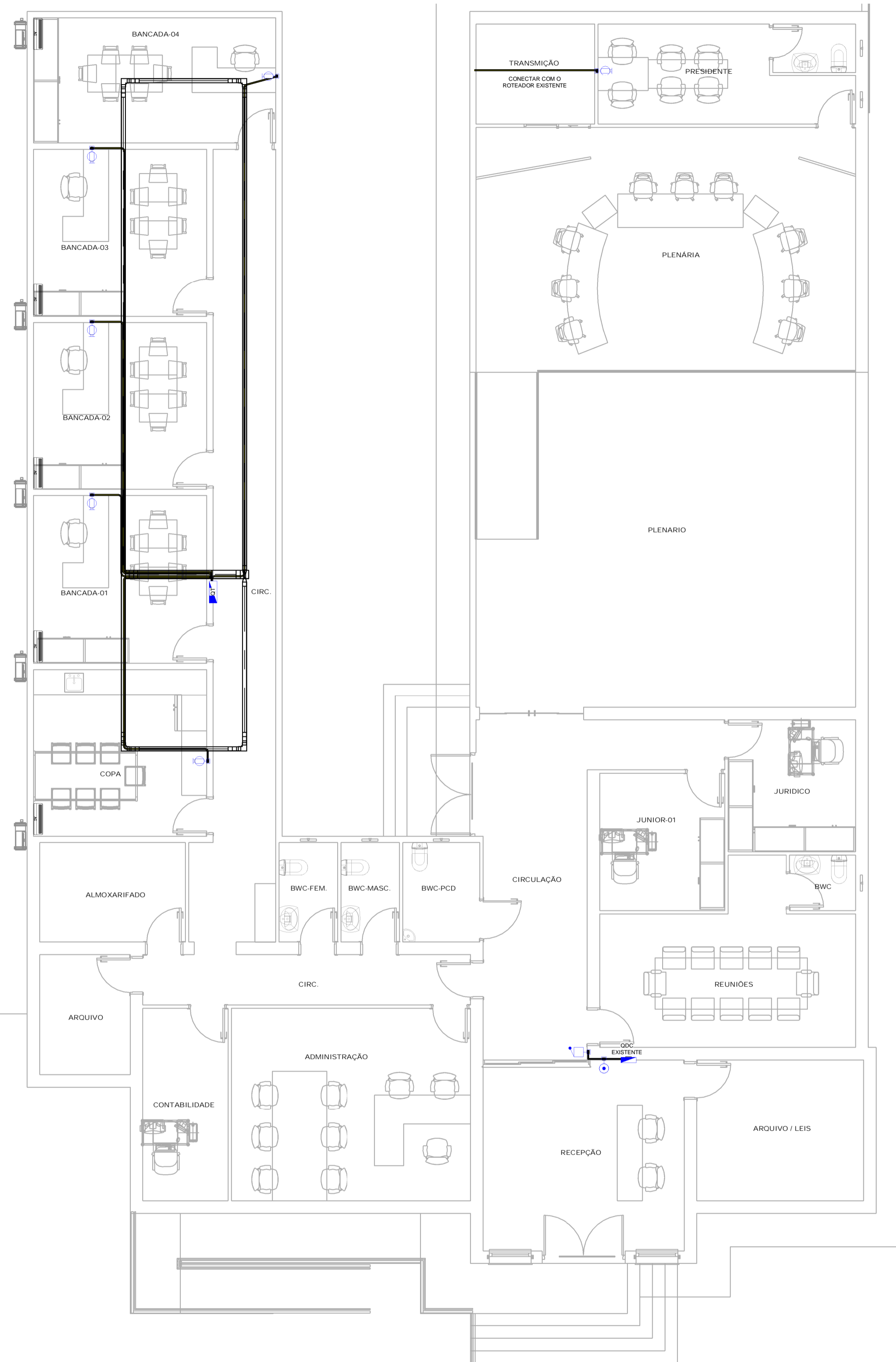
PLANTA BAIXA TELECOM ESCALA: 1:75
