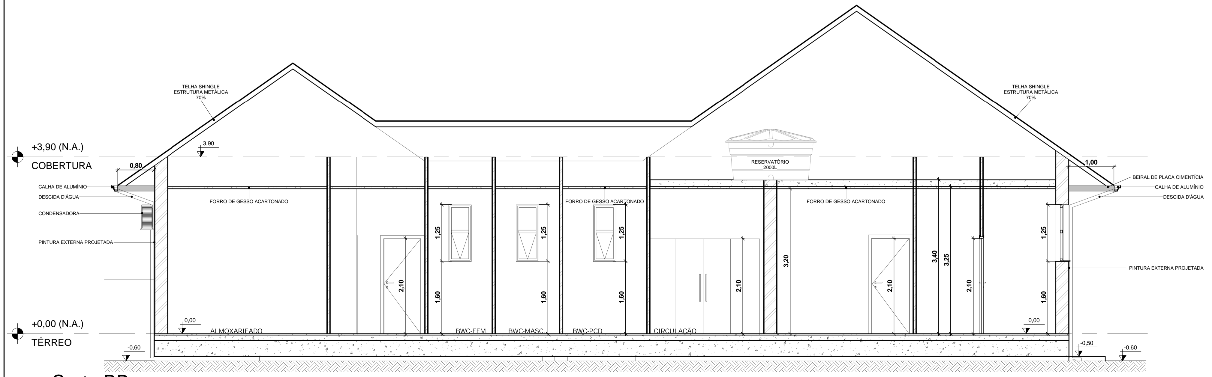
2 Corte BB 1 : 50
