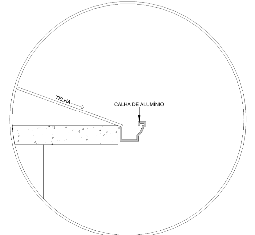
DETALHE CALHAS SEM ESCALA
