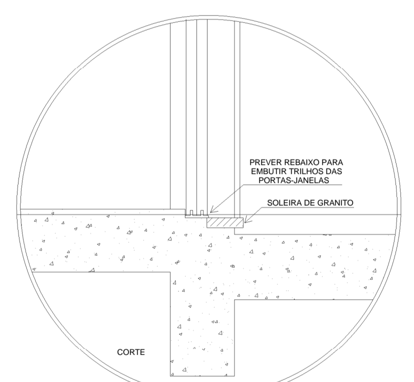
DETALHE SOLEIRA/PORTAS-JANELAS SEM ESCALA
