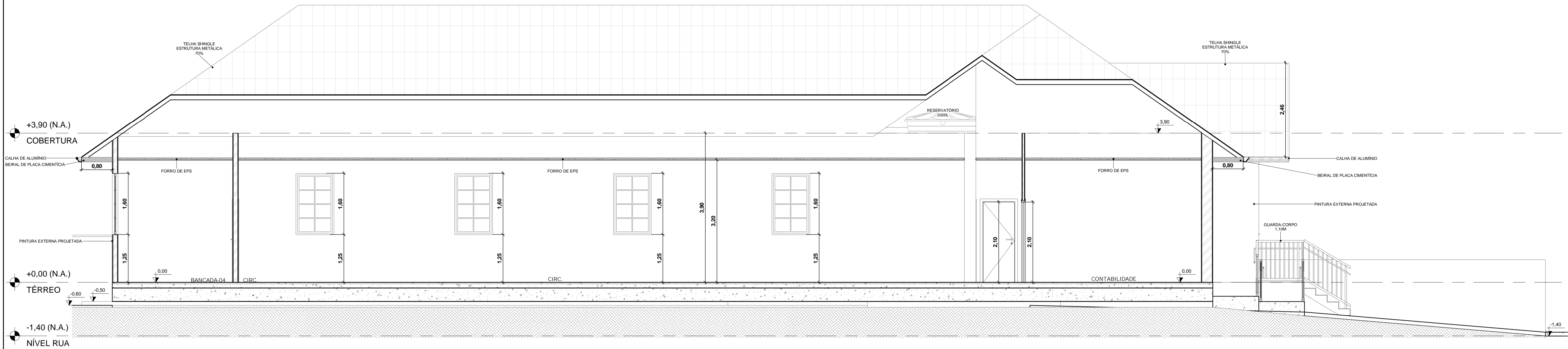
1 Corte AA 1 : 50
