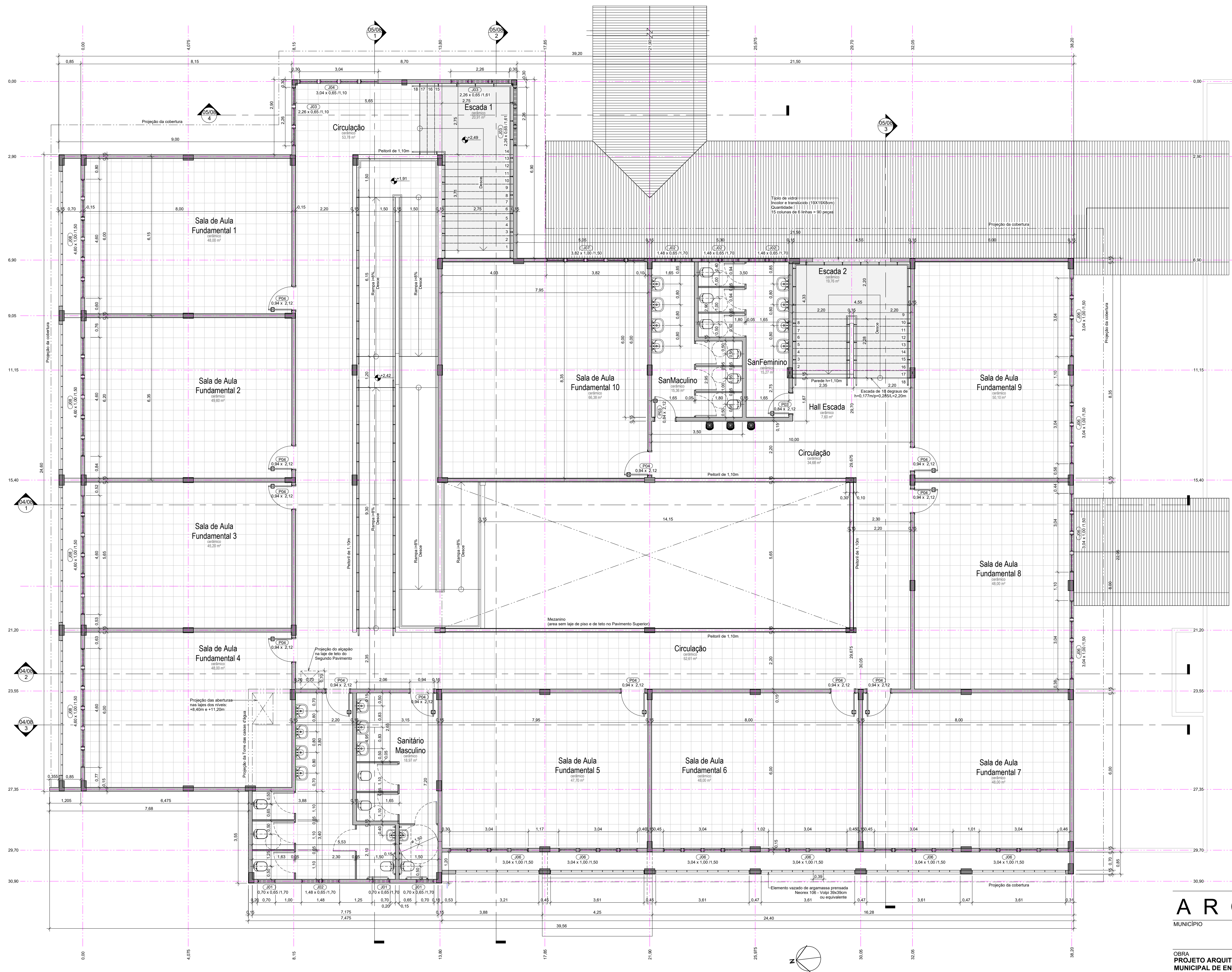
1 PLANTA BAIXA SUPERIOR Escala 1 : 75
