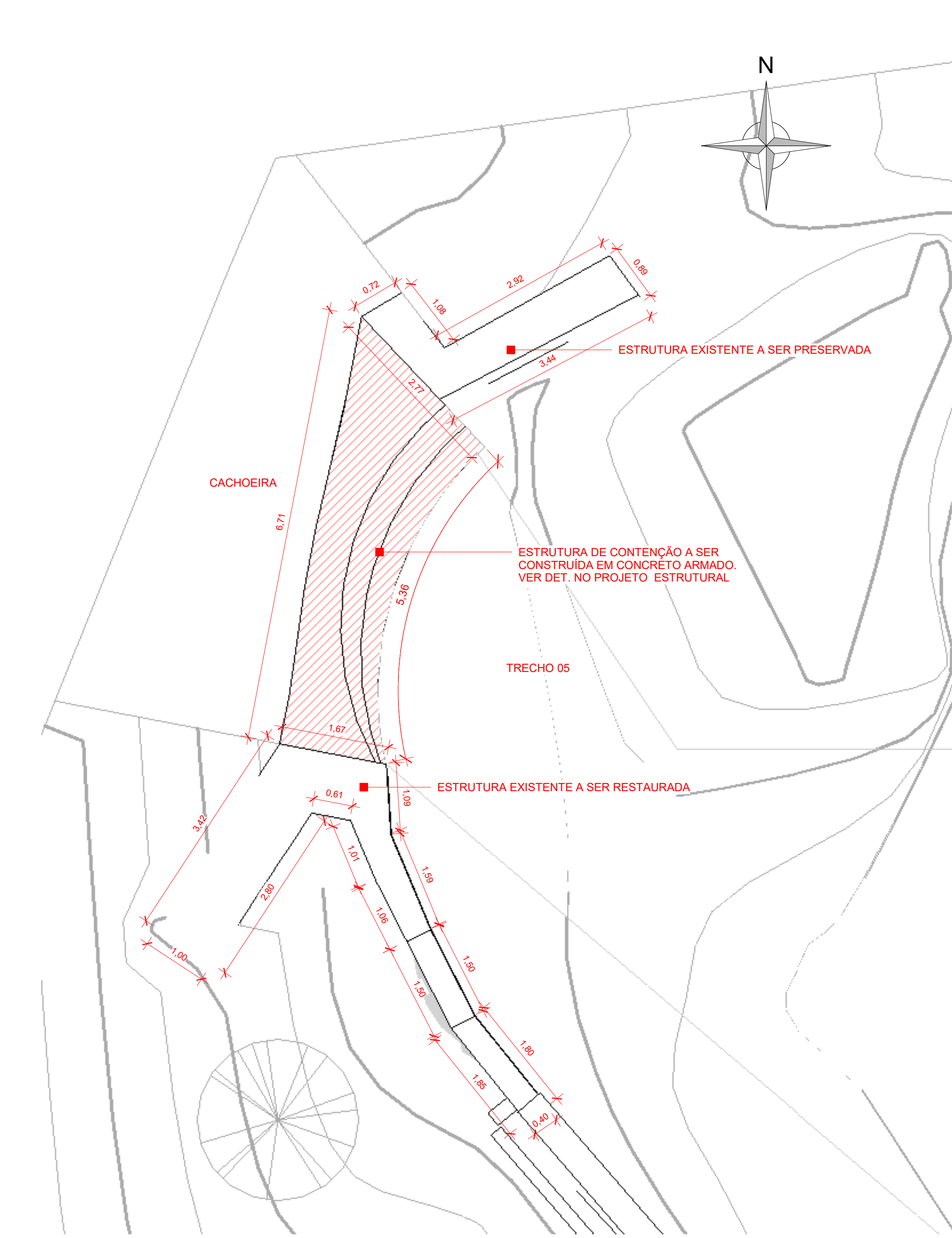
1 TRECHO 05 1 : 50
