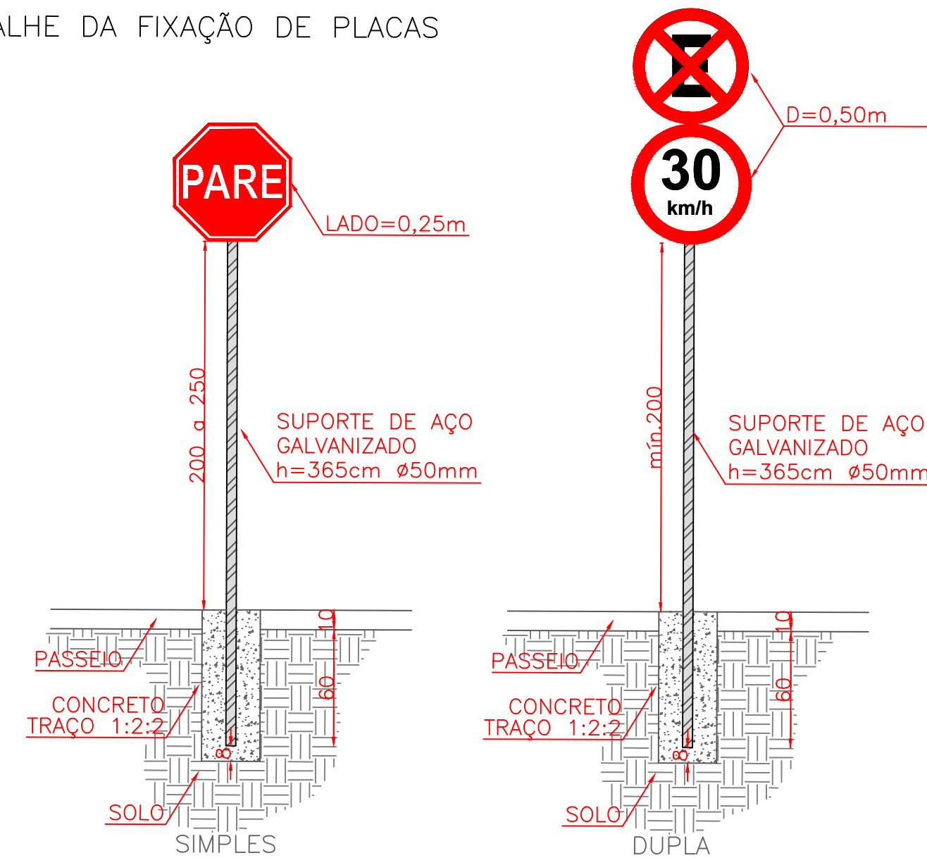
DETALHE DA FIXAÇÃO DE PLACAS
