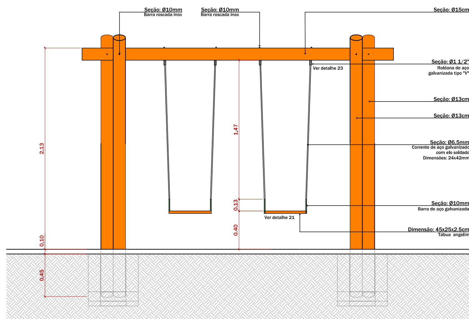
3 ELEVAÇÃO FRONTAL - BALANÇO ESCALA 1:25
