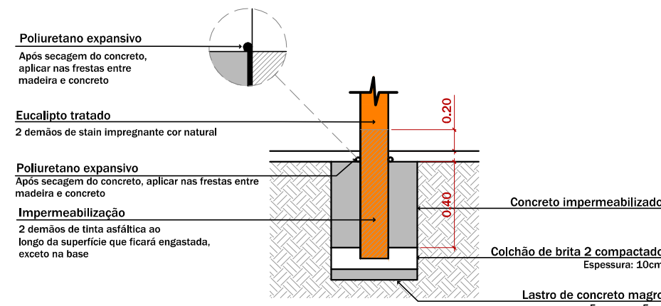
9 DETALHE - FUNDAÇÃO ACADEMIA E PLAYGROUND ESCALA 1:25
