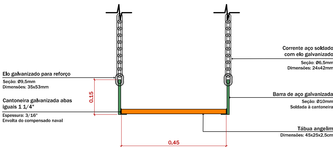
5 DETALHE - ASSENTO BALANÇO ESCALA 1:10
