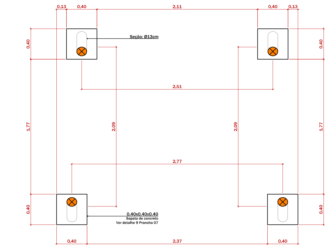
1 PLANTA NÍVEL 0 - BALANÇO ESCALA 1:25
