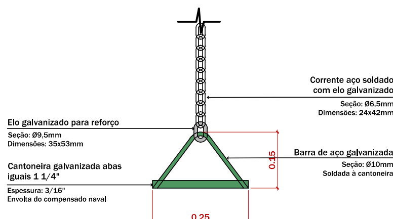
7 DETALHE - ASSENTO BALANÇO ESCALA 1:10
