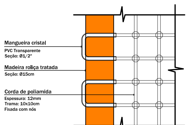
10 DETALHE - TRAMA CASTELO ESCALA 1:10
