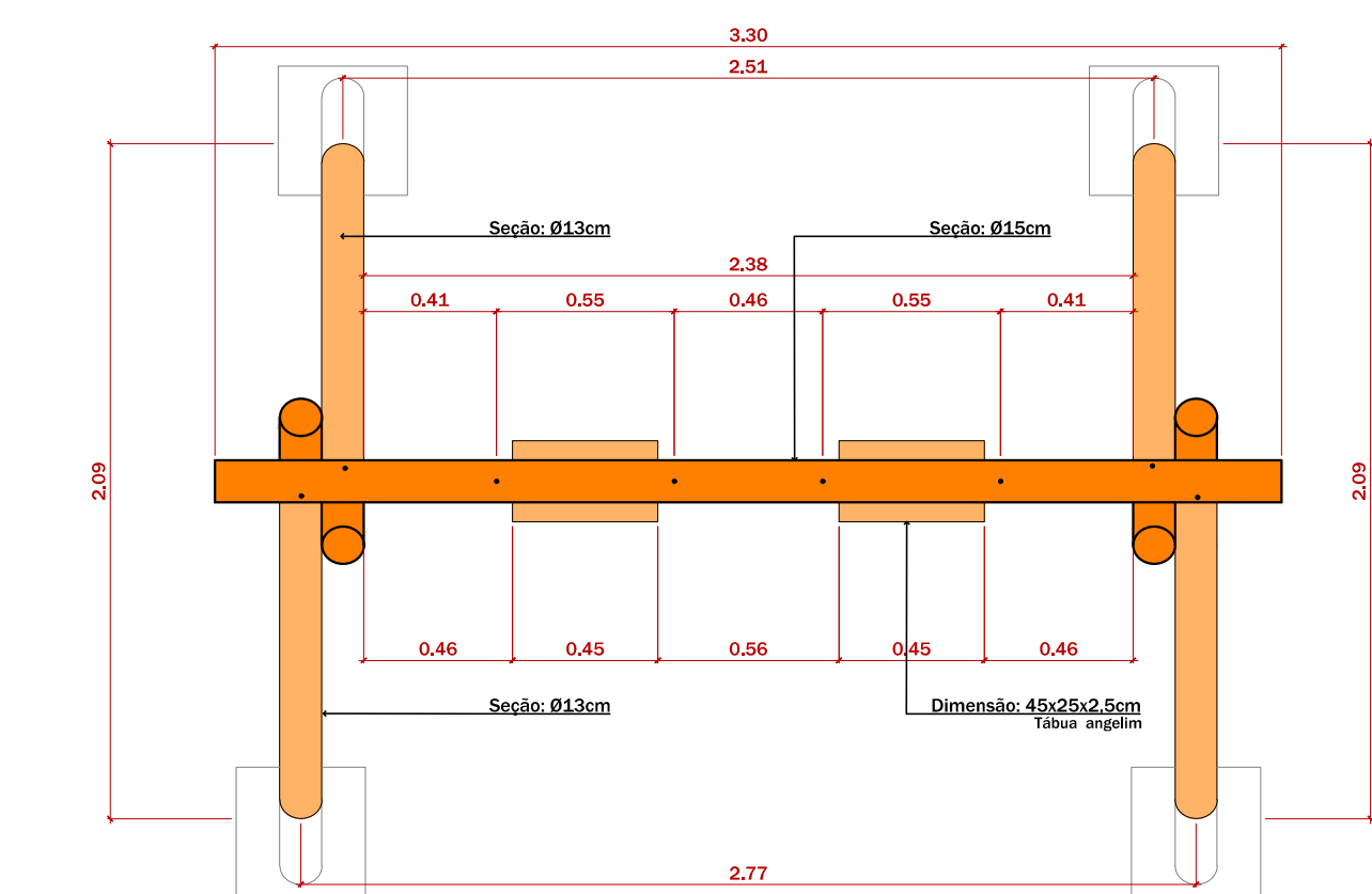
2 COBERTURA - BALANÇO ESCALA 1:25
