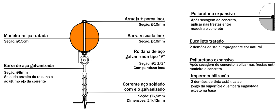
8 DETALHE - ROLDANA BALANÇO ESCALA 1:10
