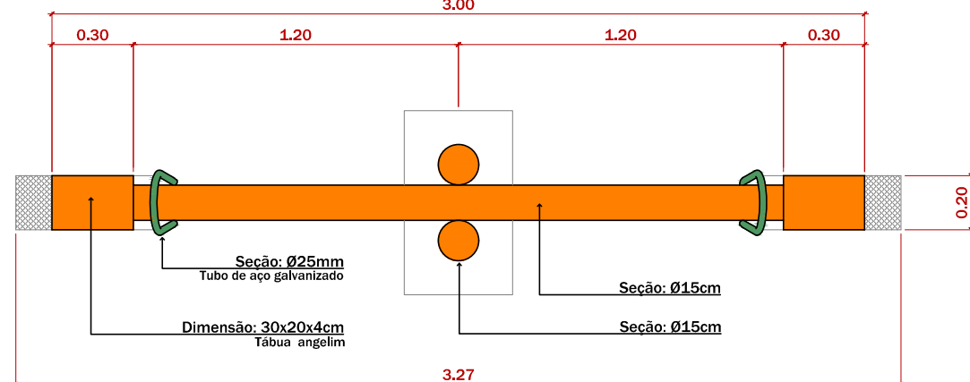
6 COBERTURA - GANGORRA ESCALA 1:25
