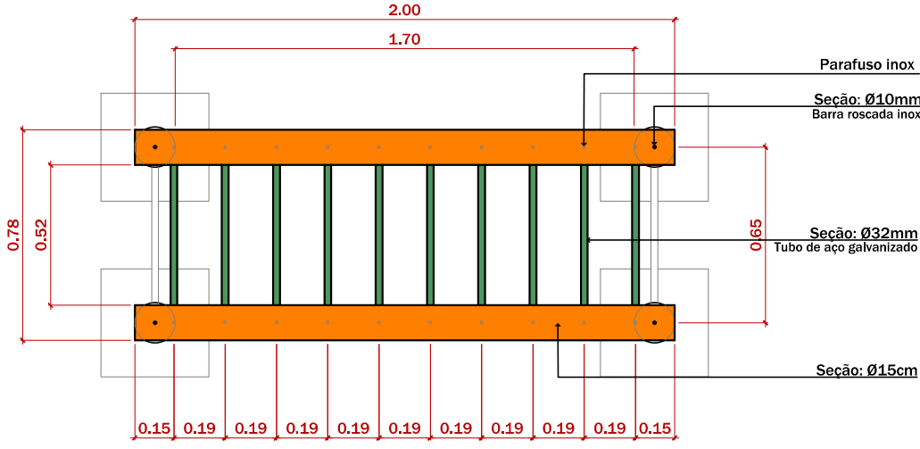
2 COBERTURA - TREPA TREPA ESCALA 1:25
