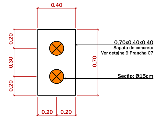
5 PLANTA NÍVEL 0 - GANGORRA ESCALA 1:25
