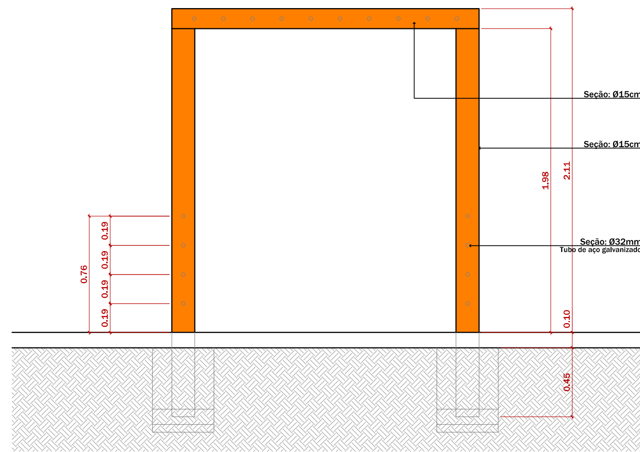
3 ELEVAÇÃO FRONTAL - TREPA TREPA ESCALA 1:25
