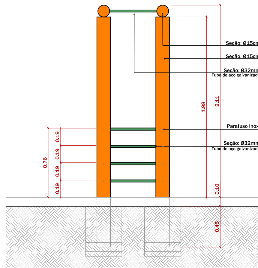
4 ELEVAÇÃO LATERAL - TREPA TREPA ESCALA 1:25
