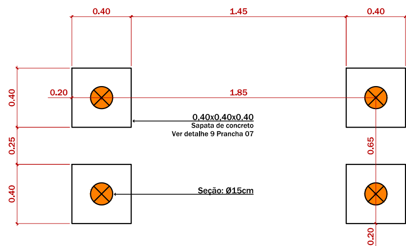
1 PLANTA NÍVEL 0 - TREPA TREPA ESCALA 1:25
