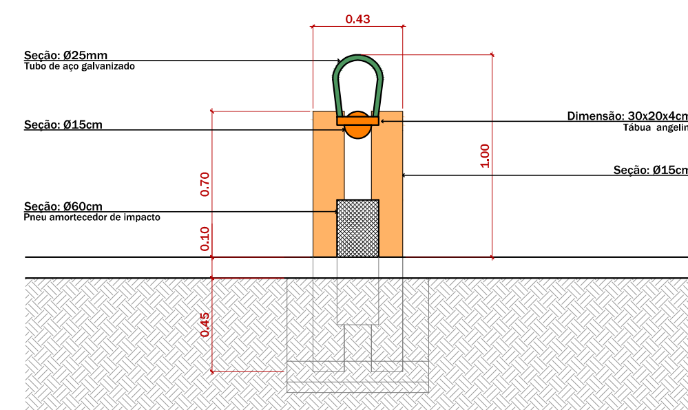
7 ELEVAÇÃO LATERAL - GANGORRA ESCALA 1:25
