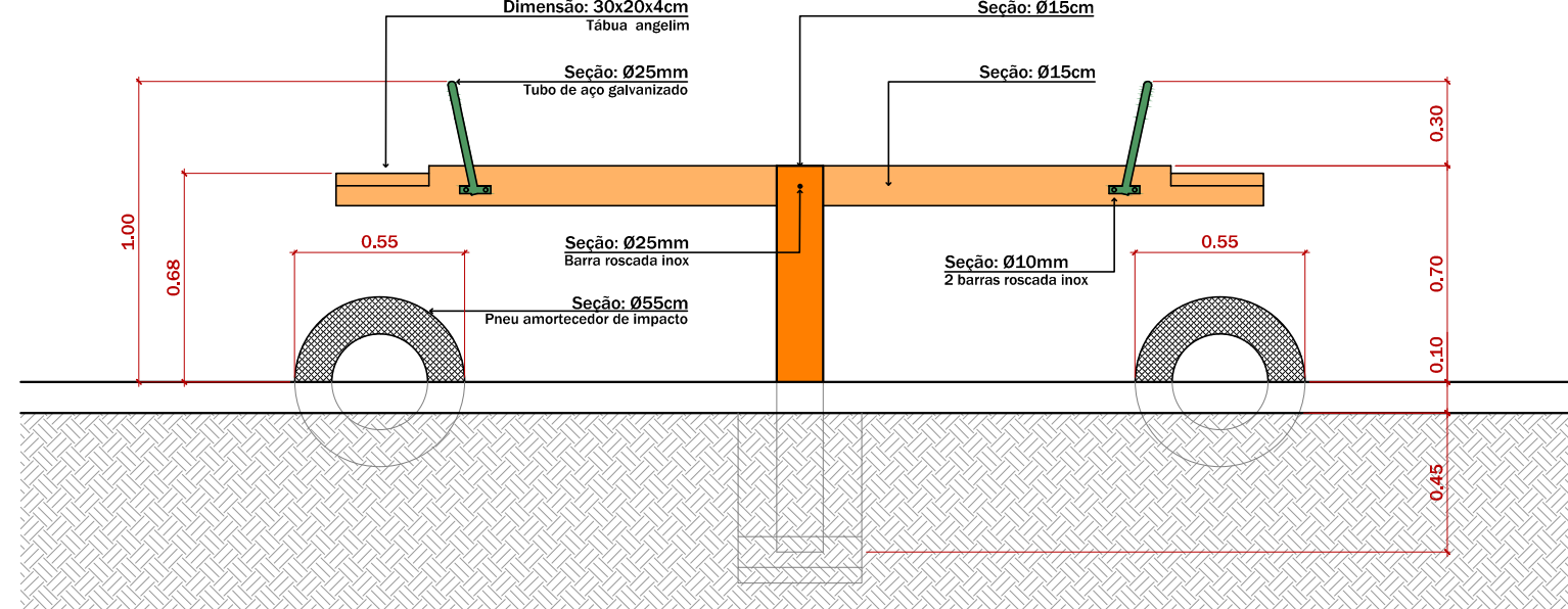
8 ELEVAÇÃO FRONTAL - GANGORRA ESCALA 1:25
