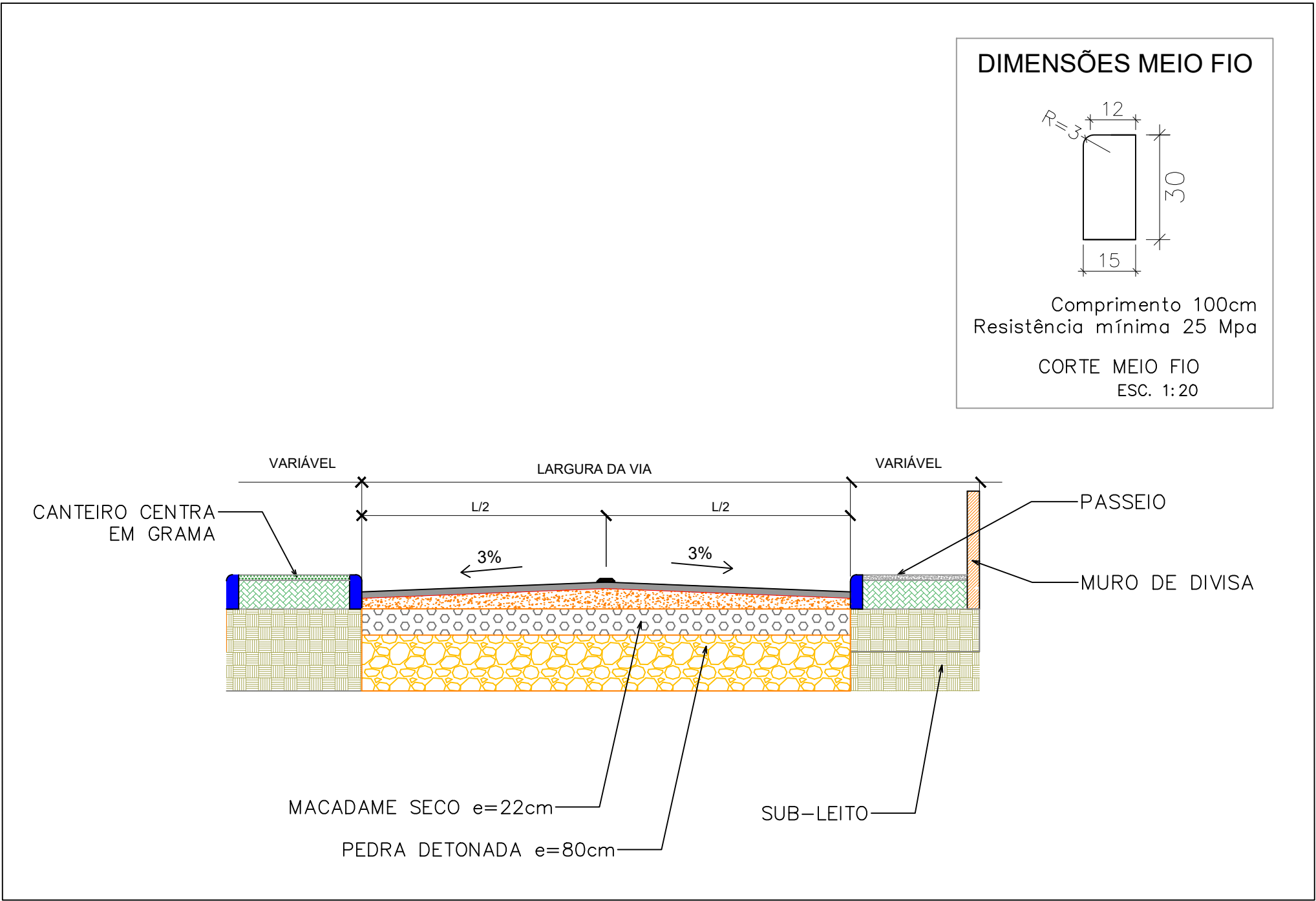
1 SEÇÃO TRANSVERSAL SEM ESCALA
