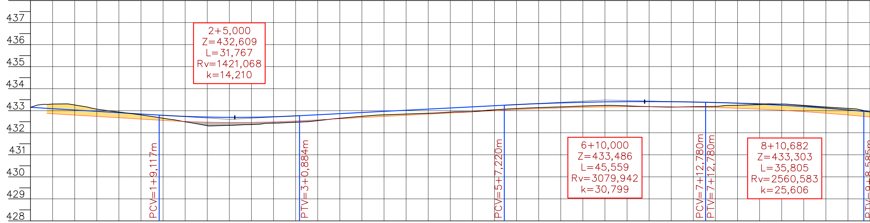
438 PERFIL LONGITUDINAL - ALINHAMENTO - Rua Pe. Daniel Henkemeier
