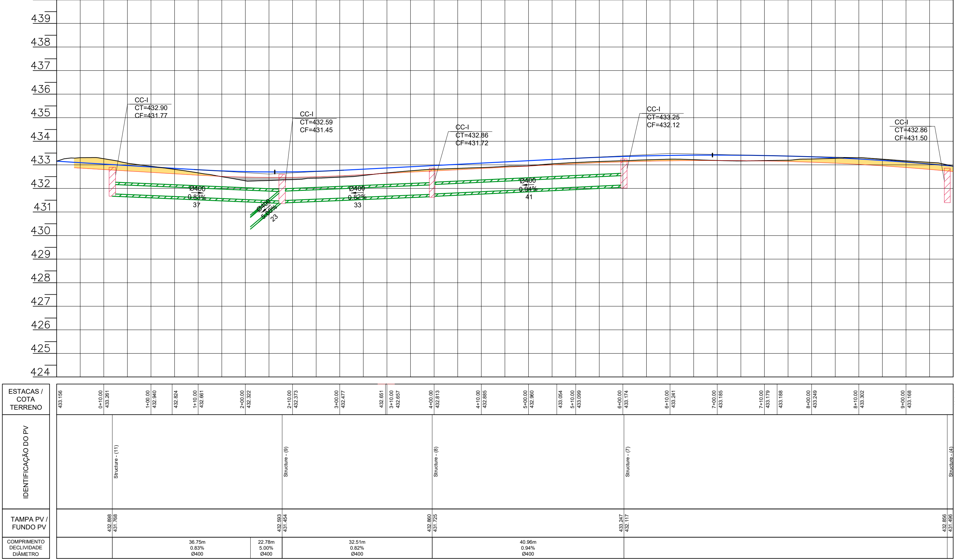
440 PERFIL LONGITUDINAL – ALINHAMENTO – Rua Pe. Daniel Hemkemeier
