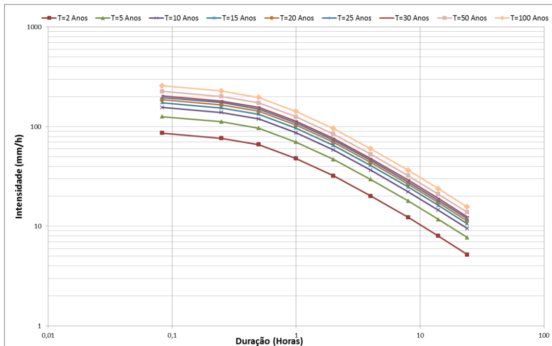
Figura 02 – Curvas intensidade-duração-freqüência
